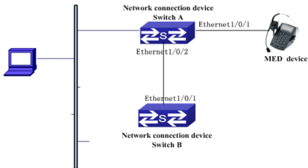
图 3-8 LLDP-MED 基本配置功能组网图
