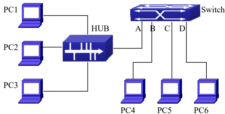
图 4-8 ARP GUARD 原理图
