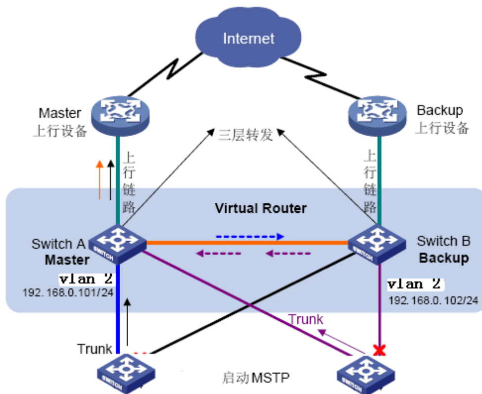
图 5-21 BFD 与 VRRP 联动
