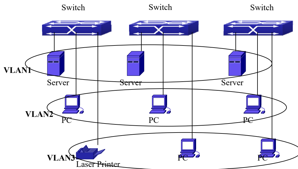
图 3-26 按照逻辑定义的 VLAN 网络
