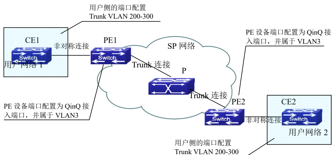
图 3-31 基于 Dot1q-tunnel 的互连模式
