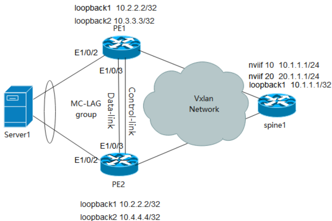
图 13-14 MC-LAG 接入集中式 VXLAN 网络配置举例
