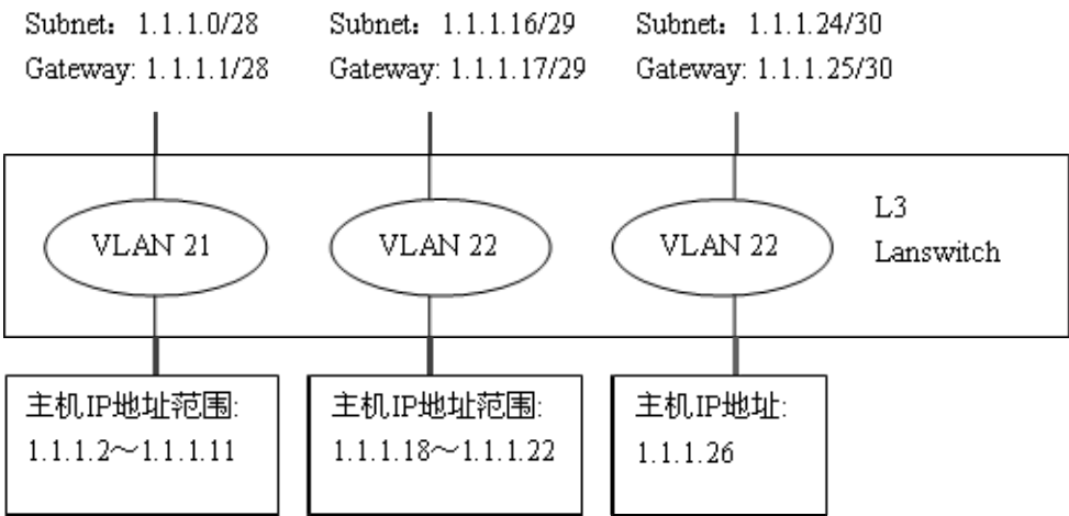
图 3-36 普通 VLAN 网络示意图
