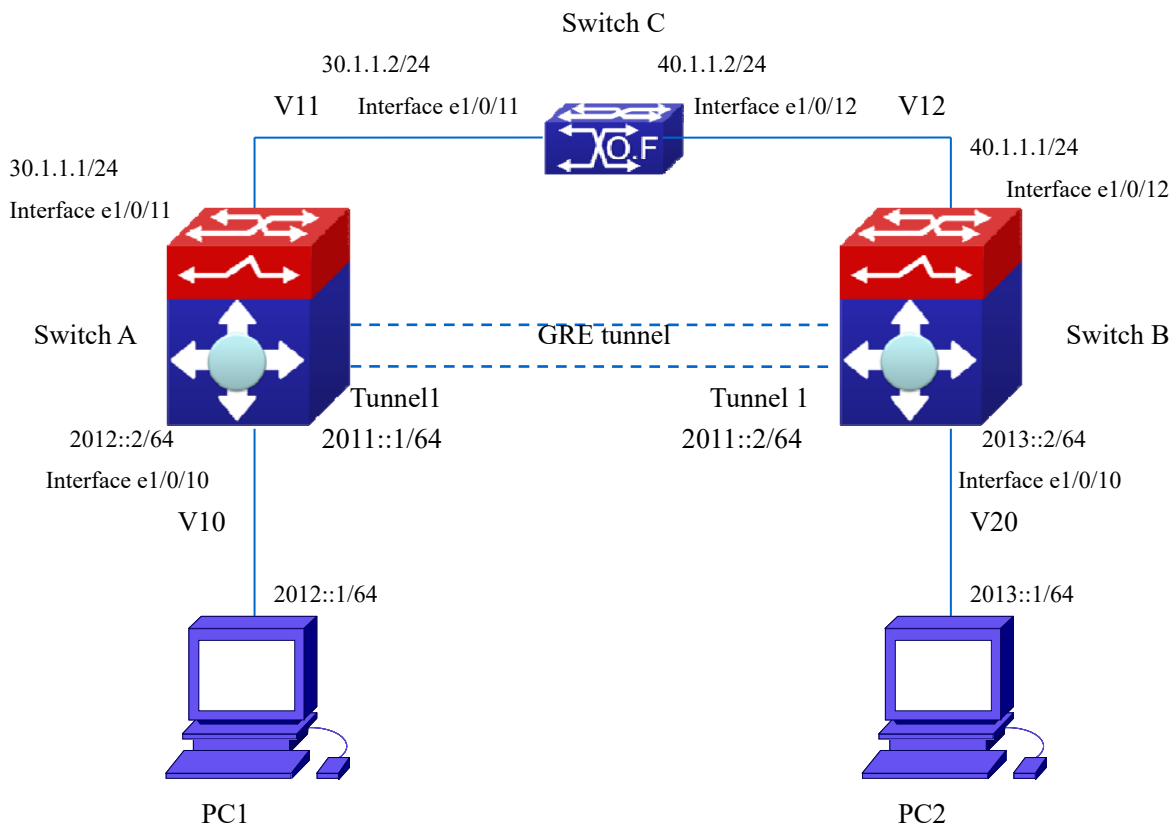
图 5-15 IPv6 over IPv4 GRE 隧道特性典型配置组网图
