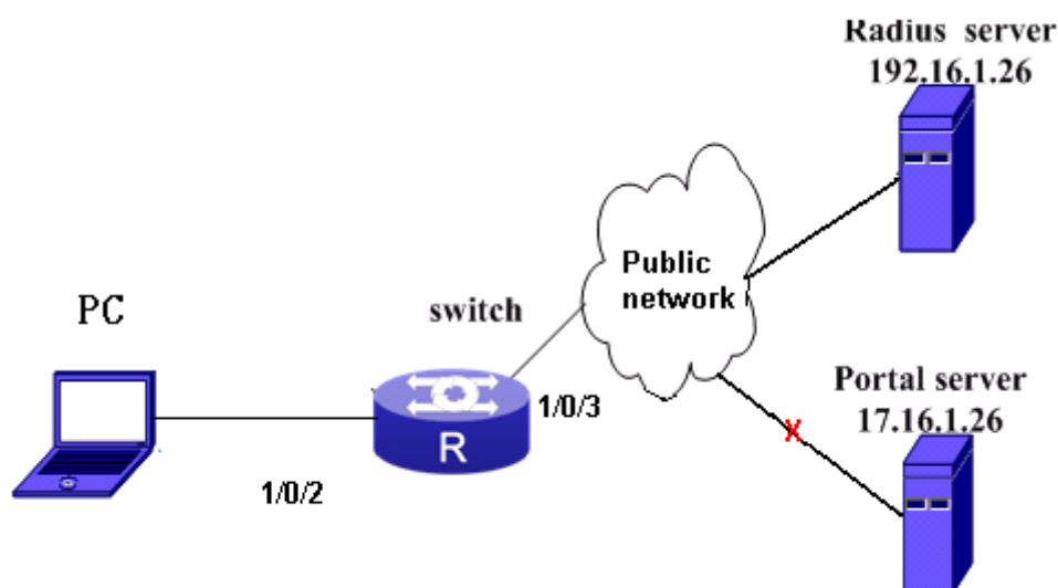
图 7-36 ortal Server 逃生功能典型案例
