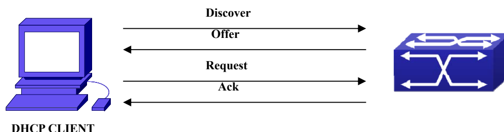
图 4-14 DHCP 协议交互过程
