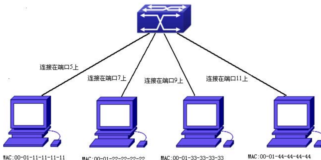
图 3-40 MAC 地址表典型配置举例
