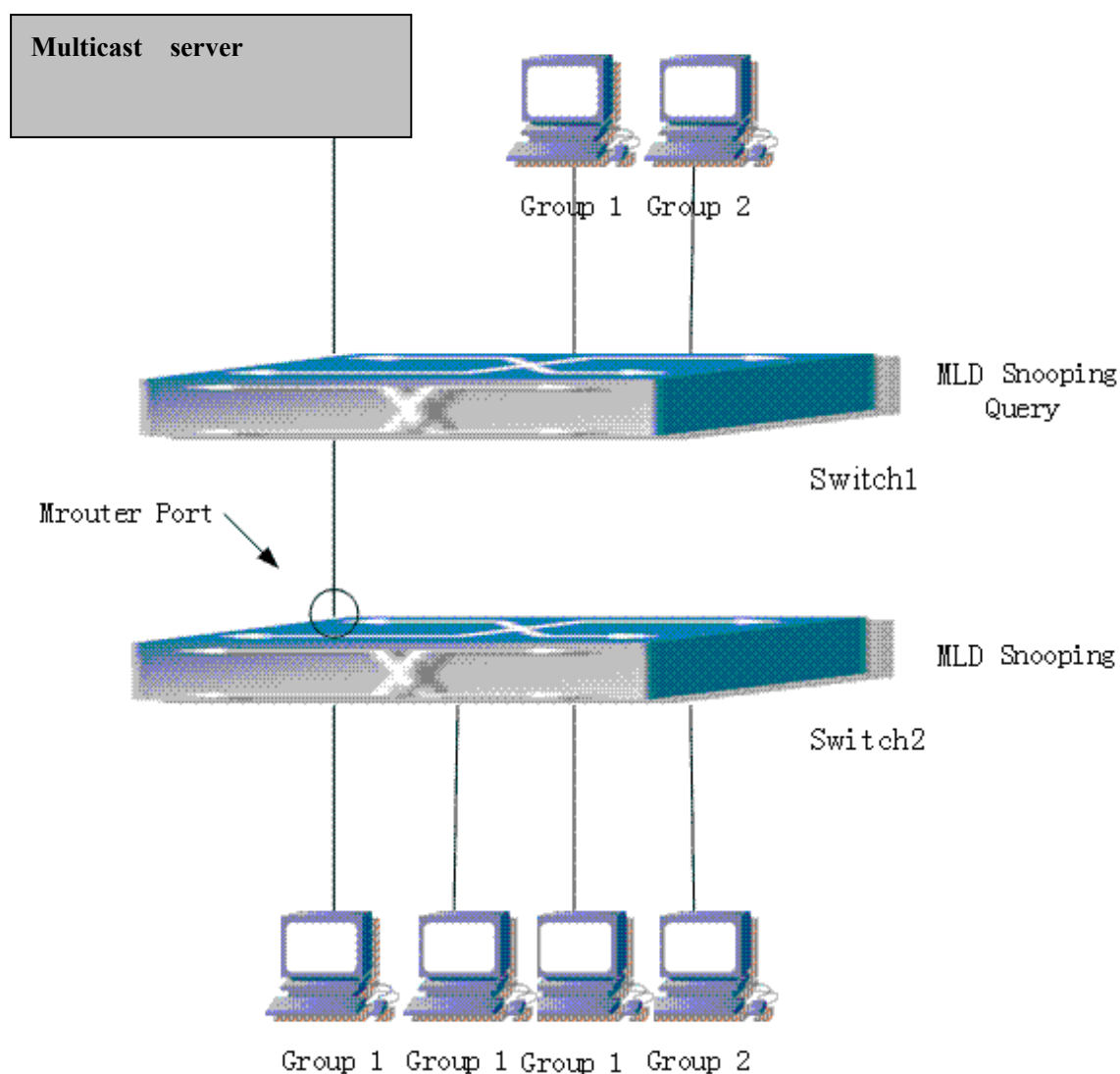
图 13-18 交换机作为 MLD Querier 功能图
