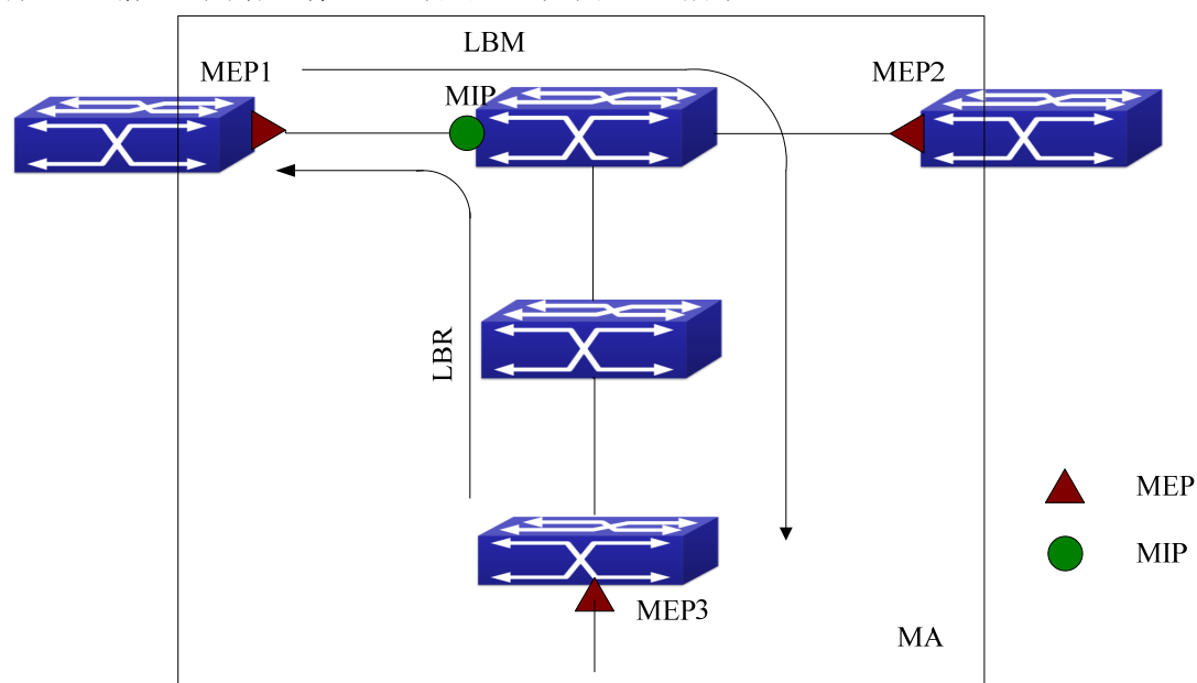
图 3-23 环回功能示意图
