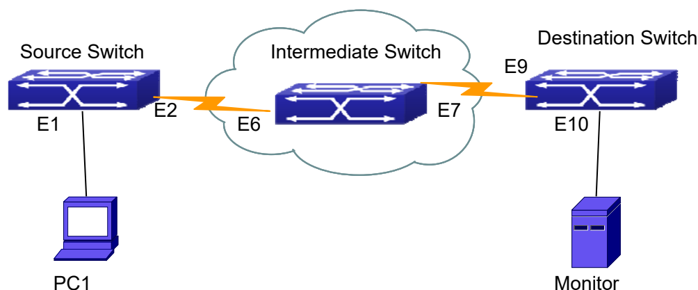
图 9-1 RSPAN 应用示意图
