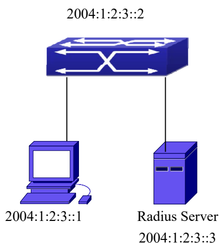
图 7-26 Pv6 Radius 配置举例拓扑图
