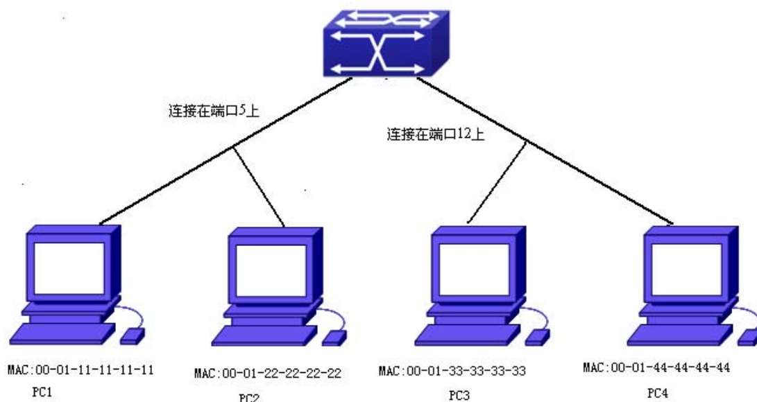
图 3-39 MAC 地址表动态学习
