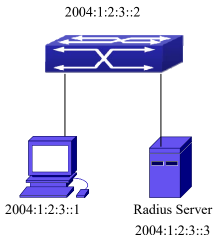
图 7-20 IPv6 Radius 配置举例拓扑图
