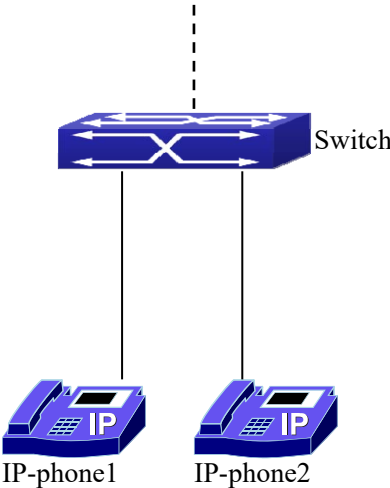
图 3-35 Voice VLAN 典型应用拓扑
