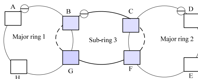
图 8-9 虚通道的交叉环拓扑
