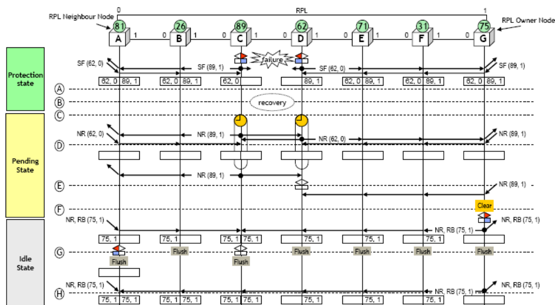
图 8-8 链路不可逆倒换方式故障恢复
