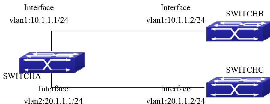
图 5-3 RIP 案例
