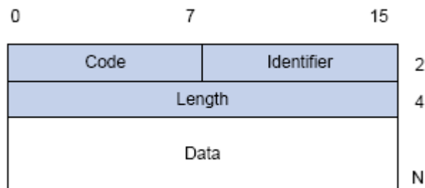
图 7-4 EAP 数据包格式
