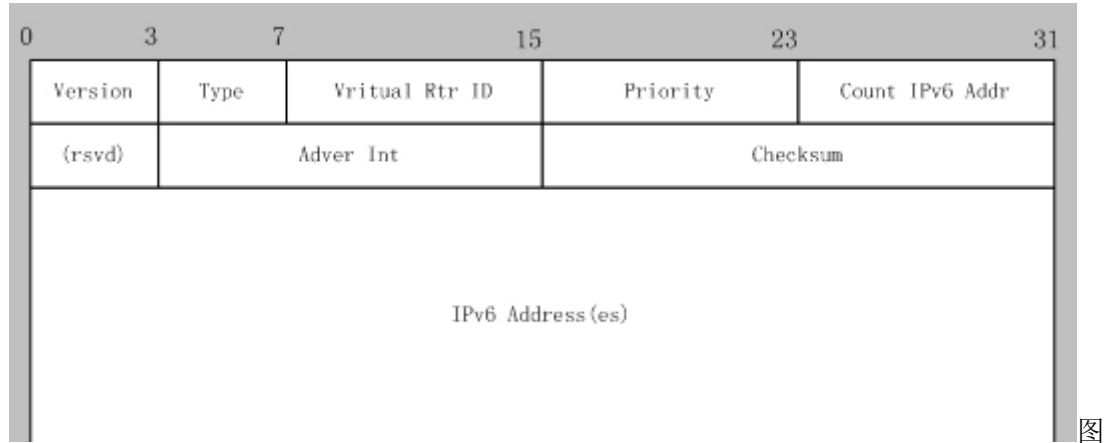
13-21 VRRPv3 报文
