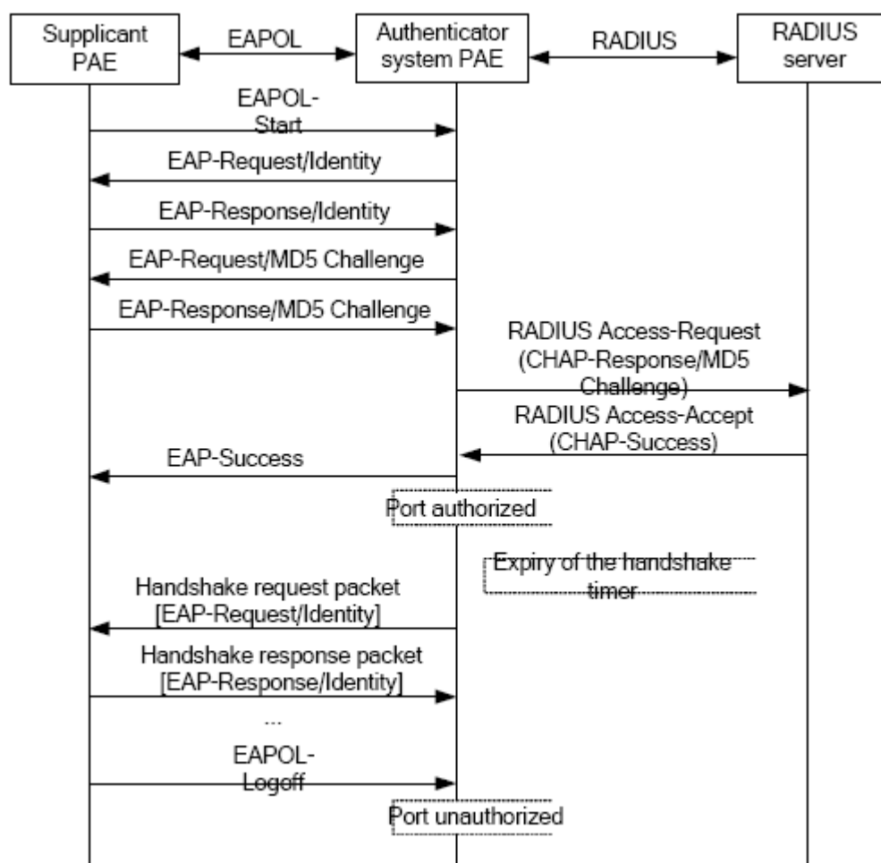
图 7-12 802.1x EAP 终结方式认证流程
