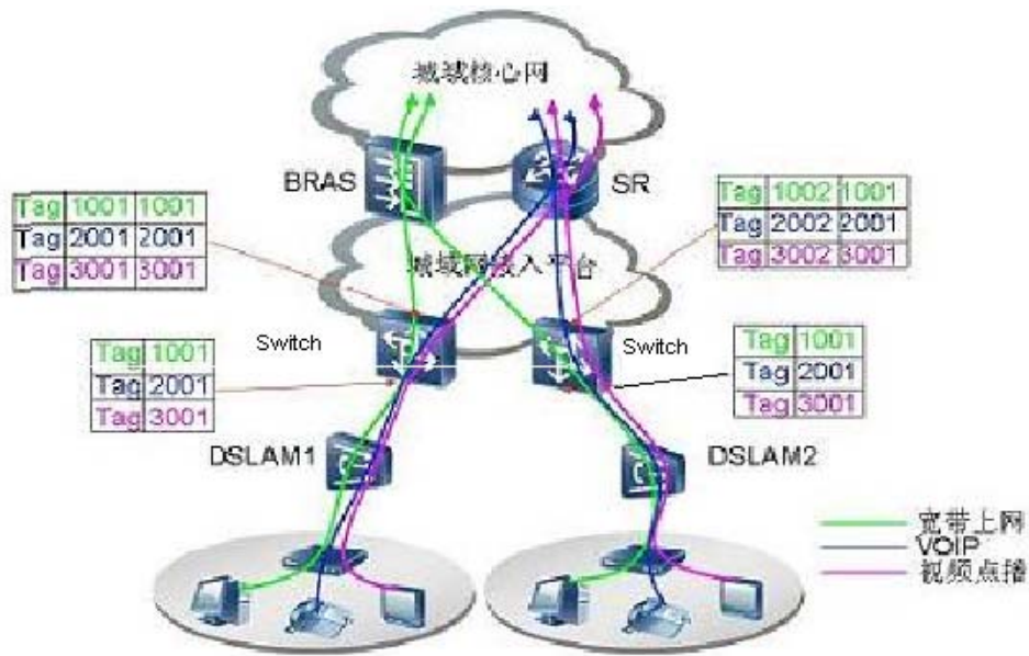
图 7-46 灵活 QinQ 应用拓扑
