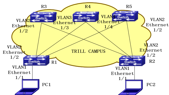
图 4-13 动态 ARP 检测功能典型案例
