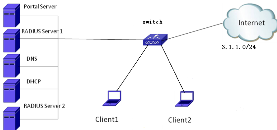
图 7-31 多 portal server 功能配置
