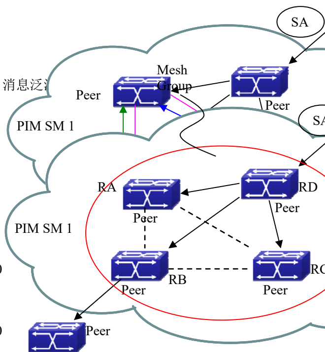
图 6-5 SA 消息泛洪
