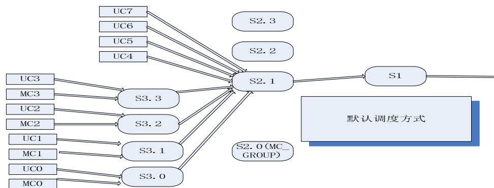
图 7-52 默认调度方式
