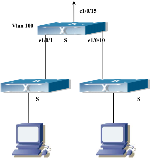
图 3-2 端口隔离功能配置案例
