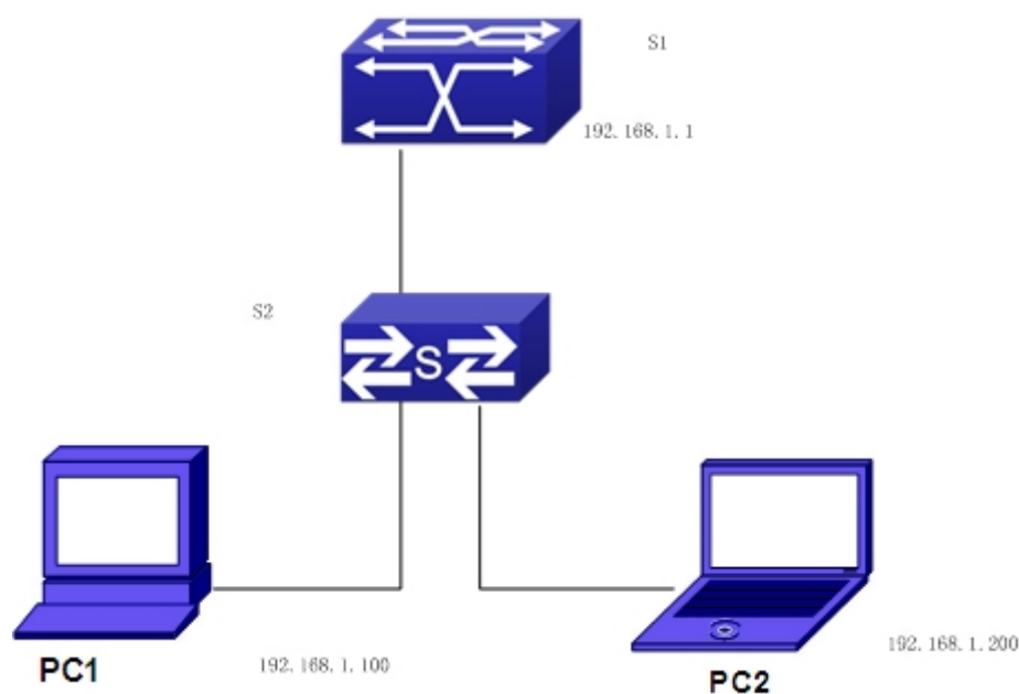
图 4-10 Arp local proxy 功能典型案例示意图
