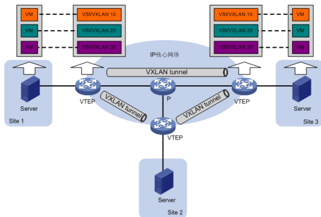
图 12-1 VXLAN 典型网络模型
