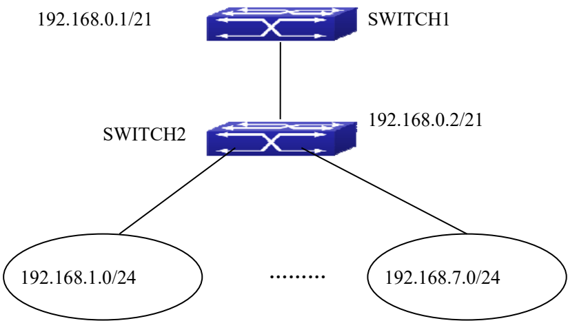
图 5-14 配置 IPv4 黑洞路由的示例图 5-59
