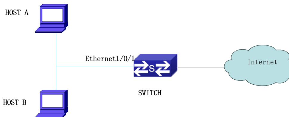
图 3-18 Port security 功能典型组网图
