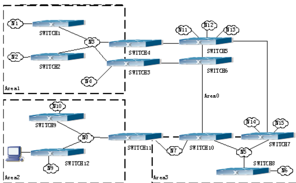
图 5-6 复杂典型 OSPF 自治系统
