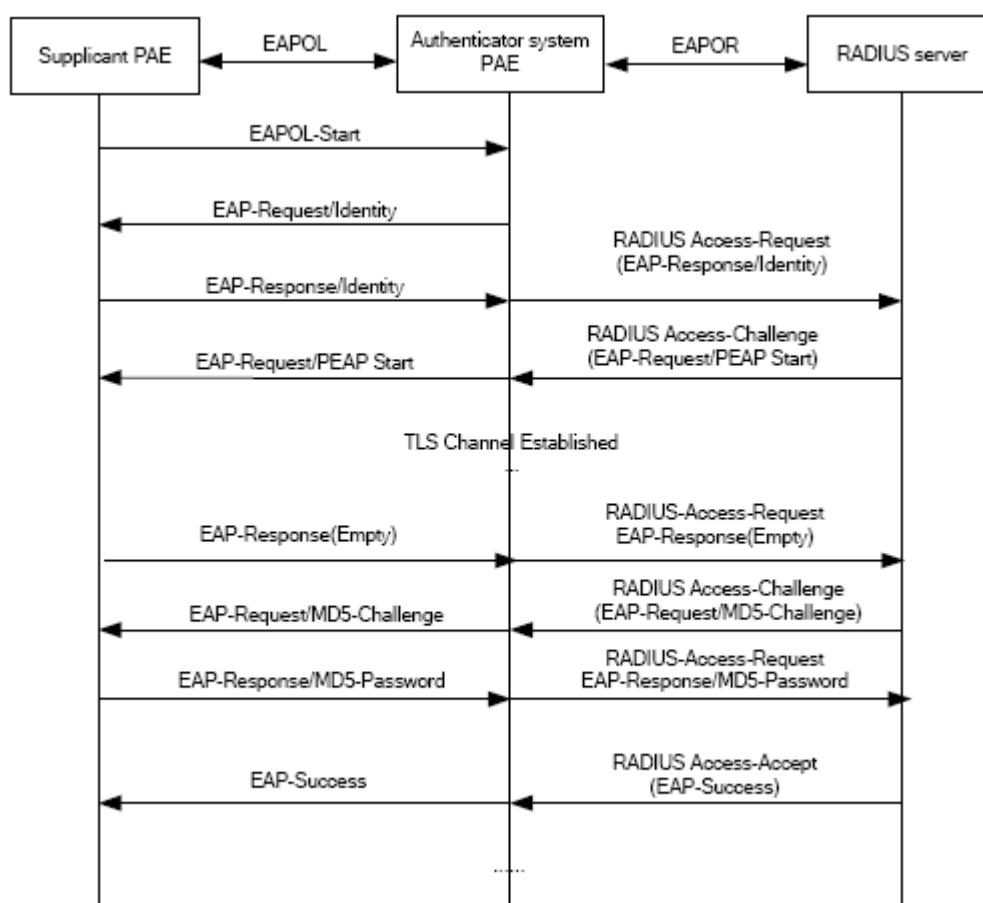
图 7-11 802.1x PEAP 认证流程
