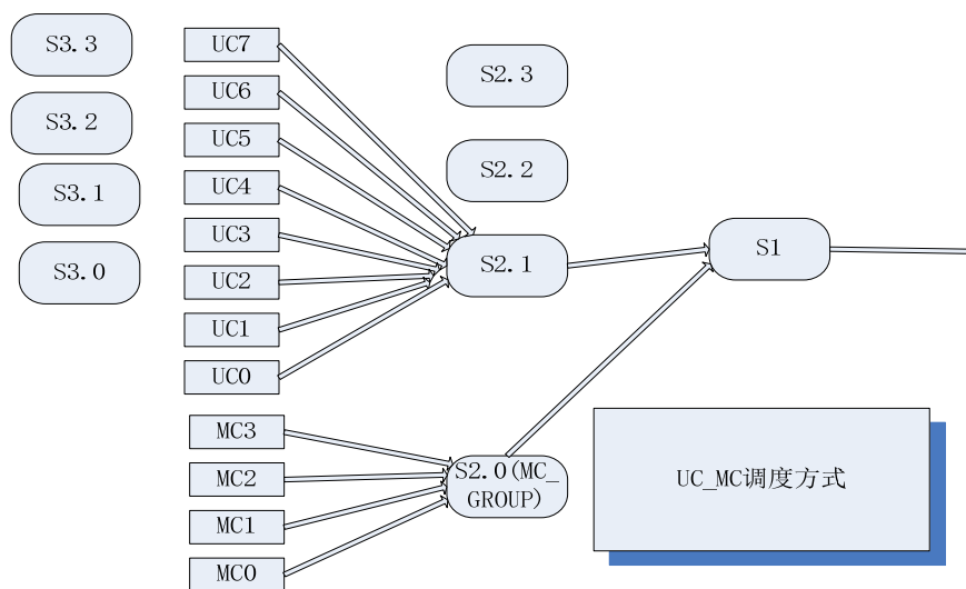
图 7-53 UC-MC 调度方式
