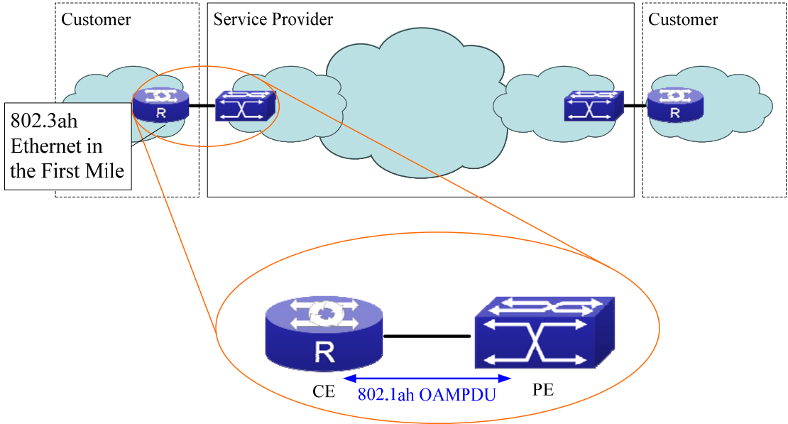
图 3-16 OAM 典型应用拓扑图
