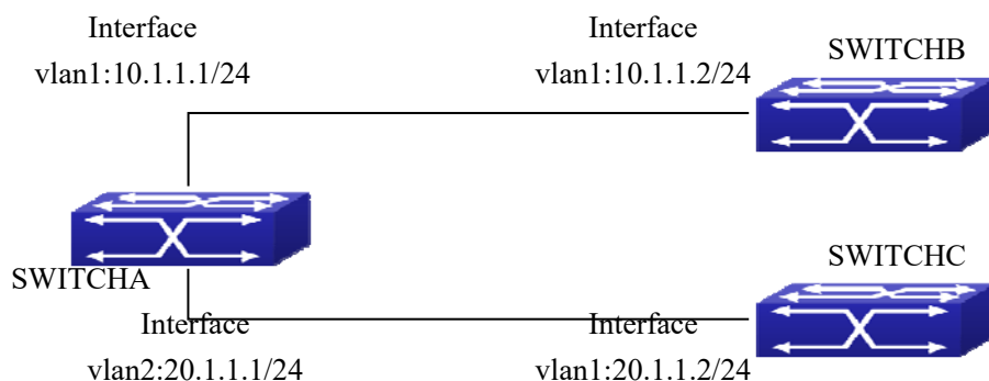
图 5-8 OSPF VPN 案例
