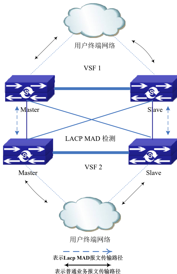
图 11-9 acp mad 检测典型拓扑
