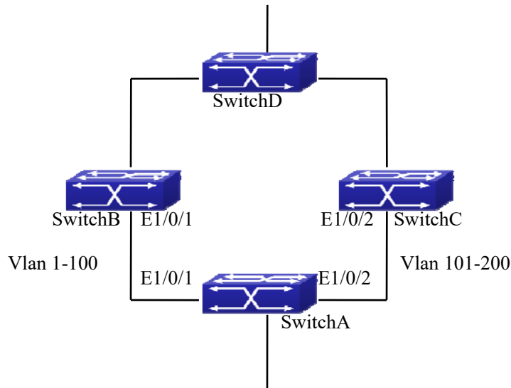
图 8-18 LPP 典型配置案例 2
