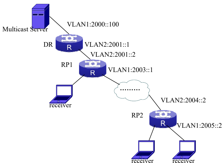
图 13-14 路由器 ANYCAST RP v6 功能
