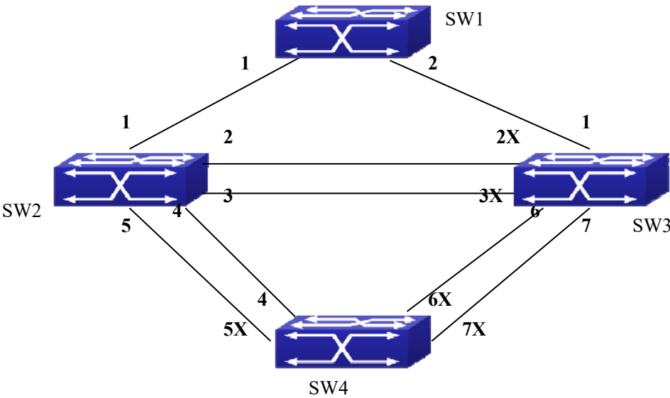
图 8-2 MSTP 典型配置举例
