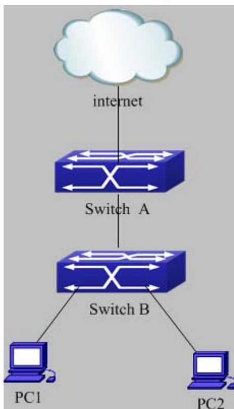
图 3-28 Hybrid 口的典型应用场景
