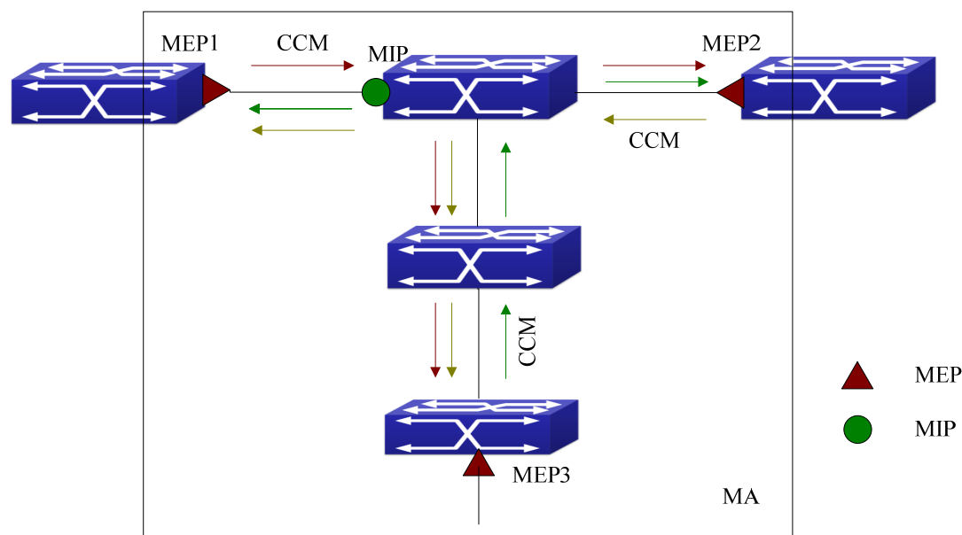
图 3-21 连通性检测示意图
