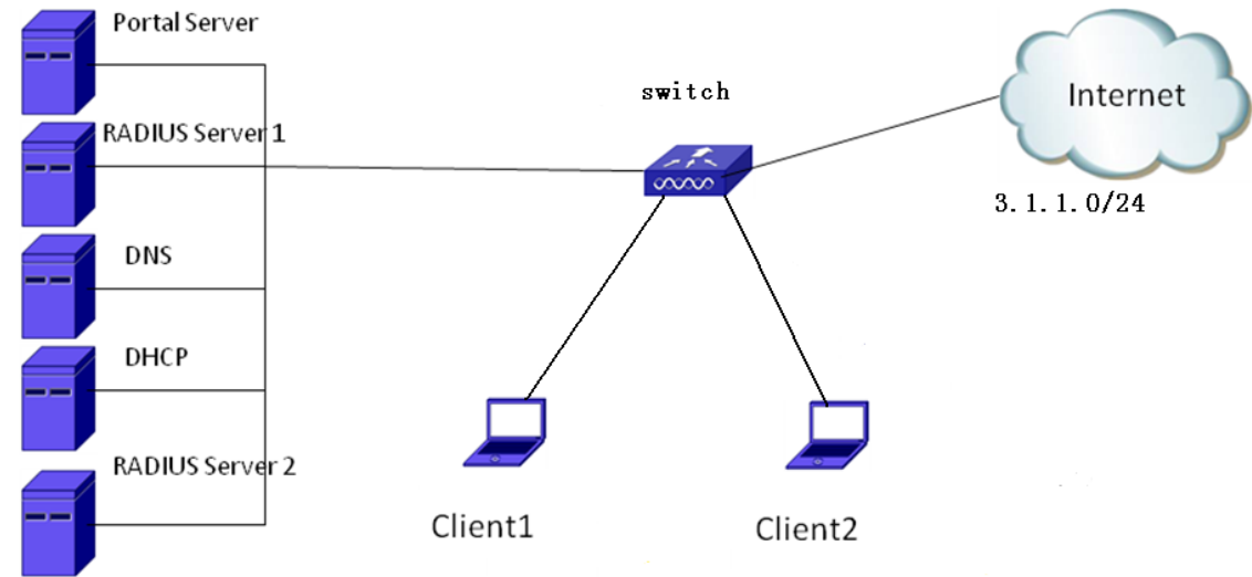
图 7-32 认证白名单功能配置图
