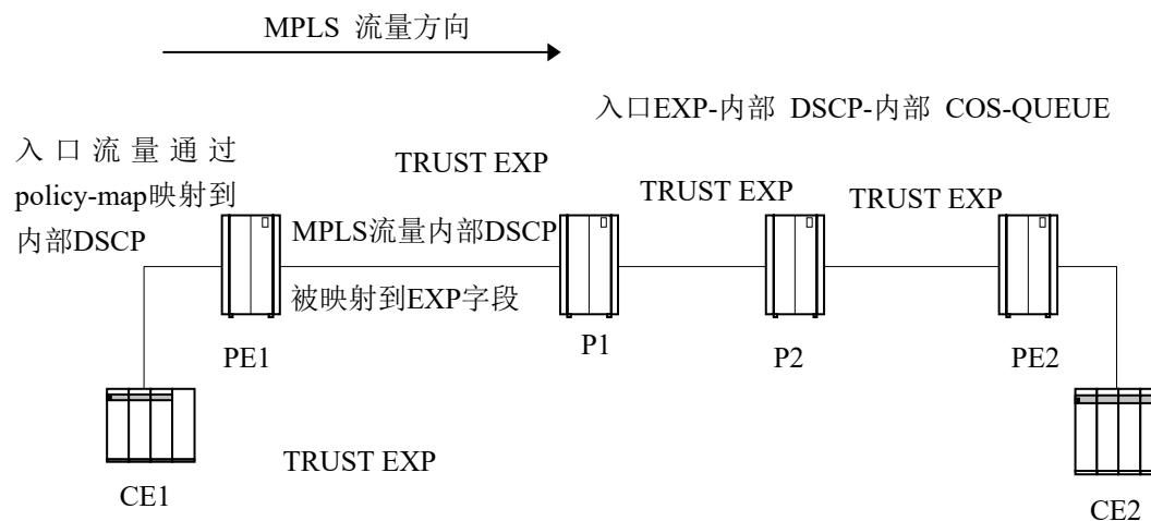
图 7-50 MPLS QoS 举例
