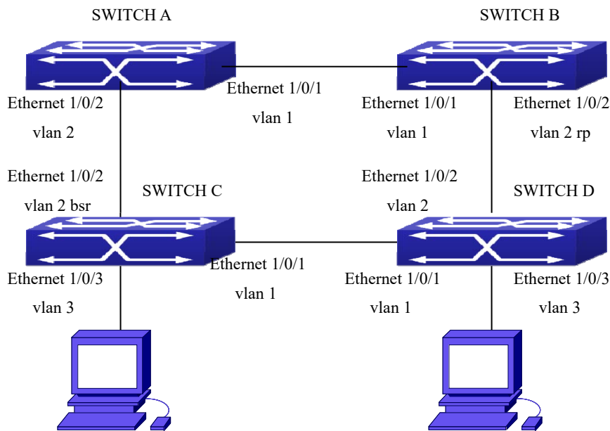
图 13-15 PIM-SSM 典型环境
