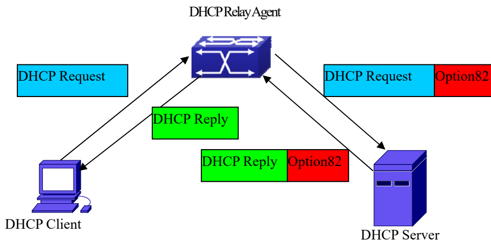
图 4-18 DHCP option 82 流程图
