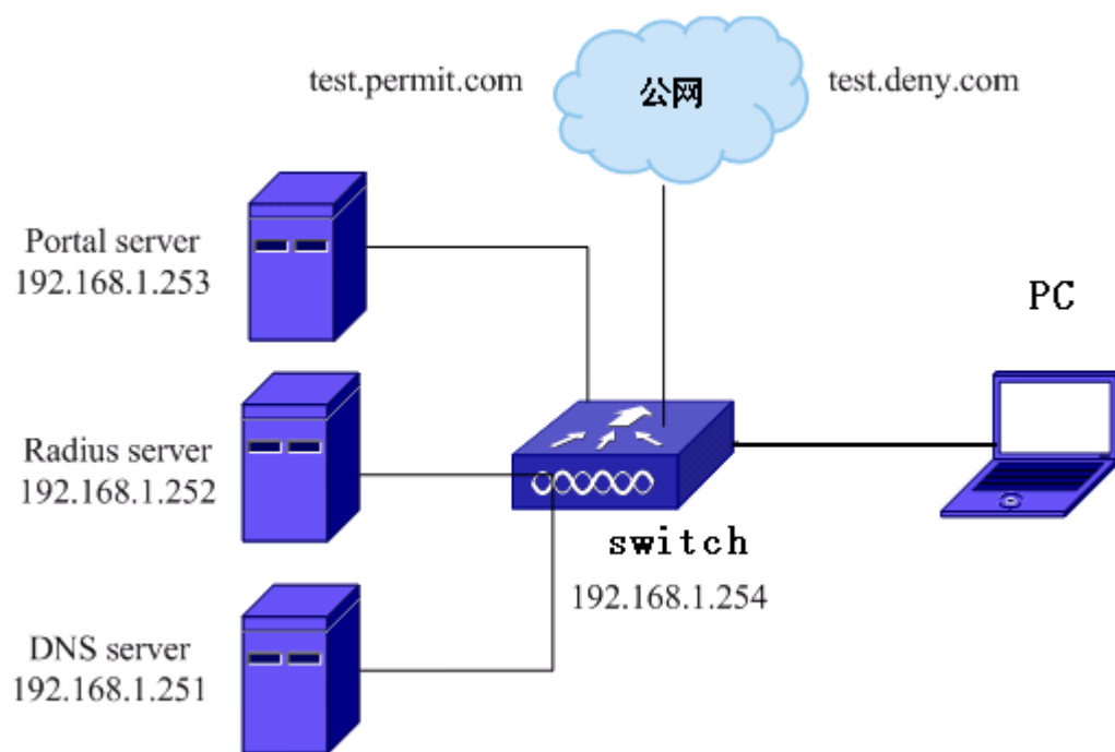
图 7-34 ttp-redirect-filter 功能典型案例
