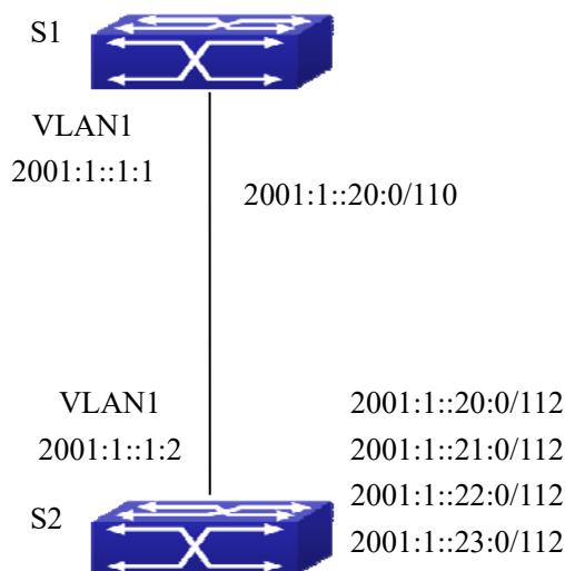
图 13-8 RIPng 路由聚合典型应用环境
