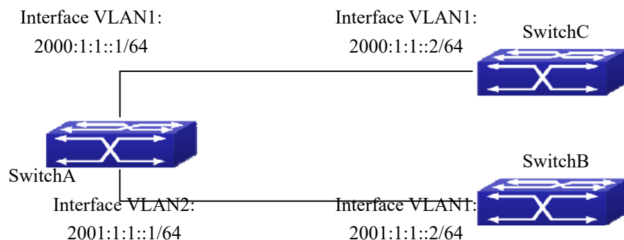
图 13-7 RIPng 案例
