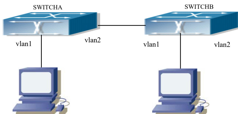
图 6-1 PIM-DM 典型环境
