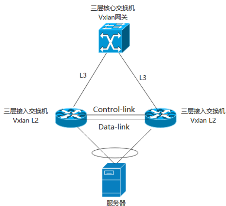
图 13-12 MC-LAG 接入 VXLAN 网络
