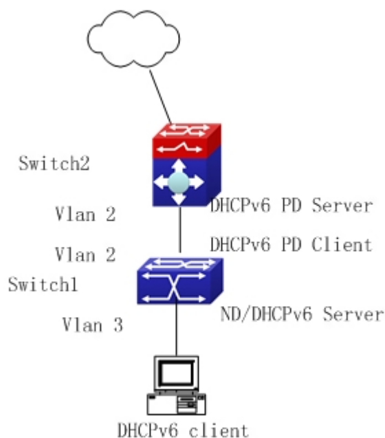
图 13-4 DHCPv6 配置举例示意图 2
