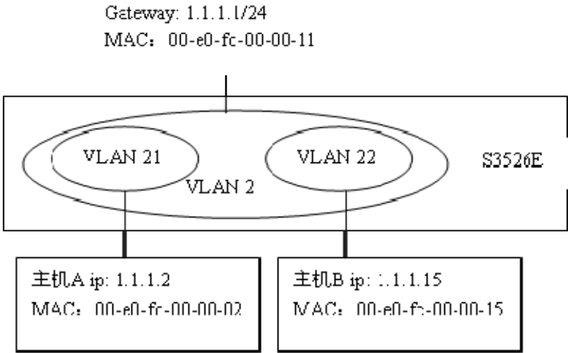
图 3-37 super vlan 功能示意图
