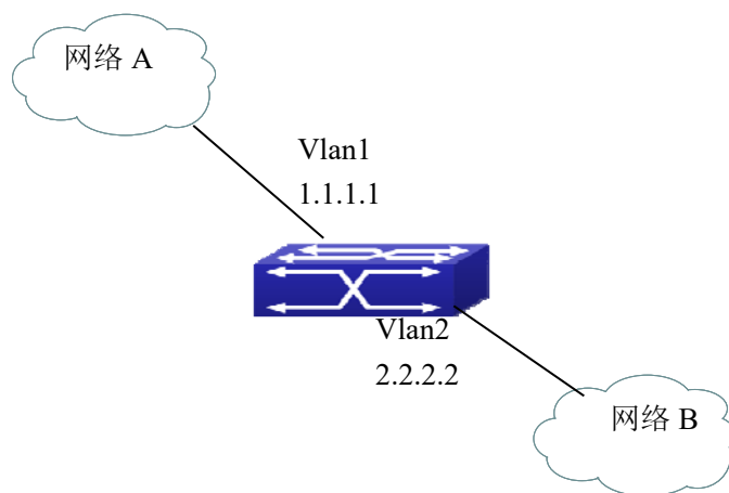
图 5-7 OSPF 引入其他 OSPF 进程路由功能案例
