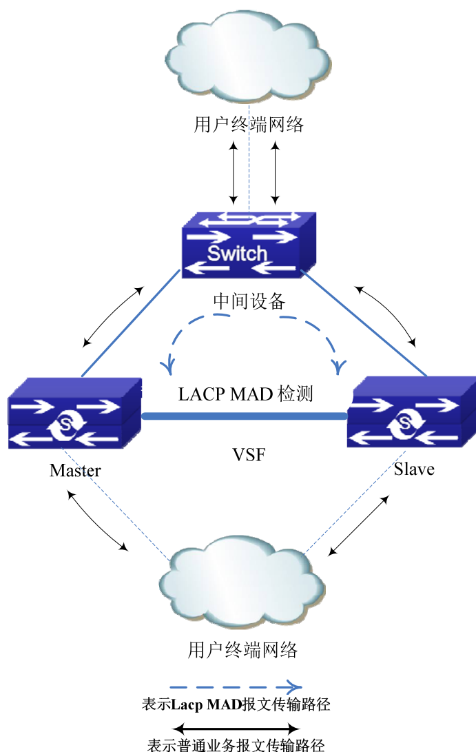
图 11-7 ACP MAD 检测
