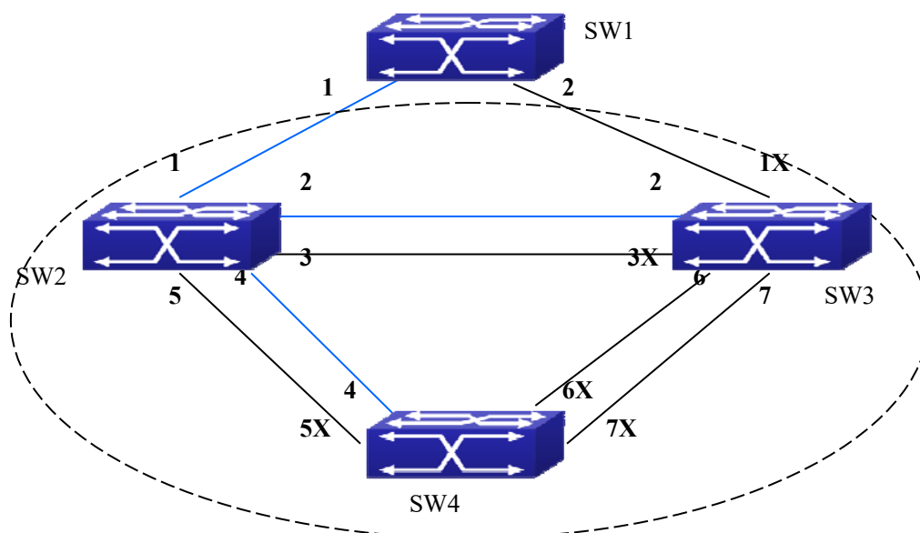
图 8-3 MSTP 变更后的实例 0 的拓扑
