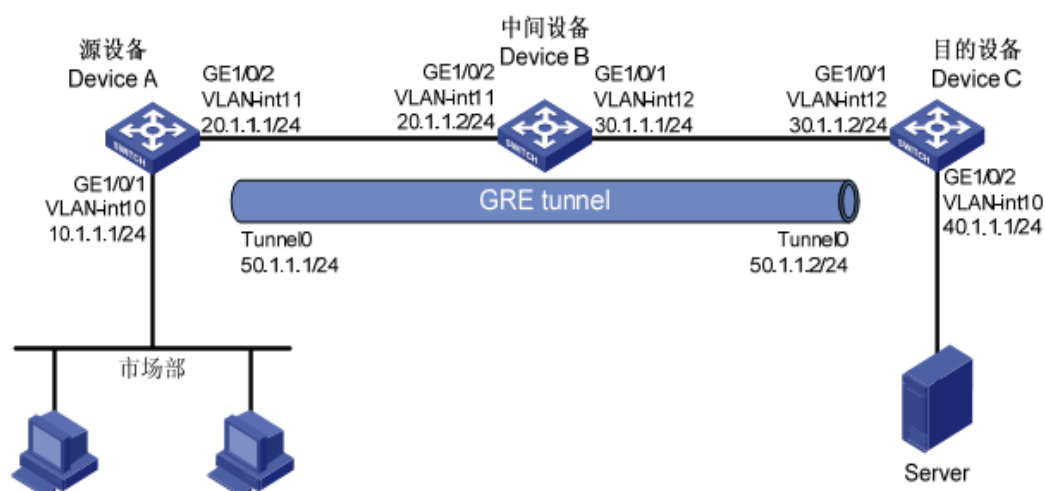
图 9-2 ERSPAN 应用示意图
