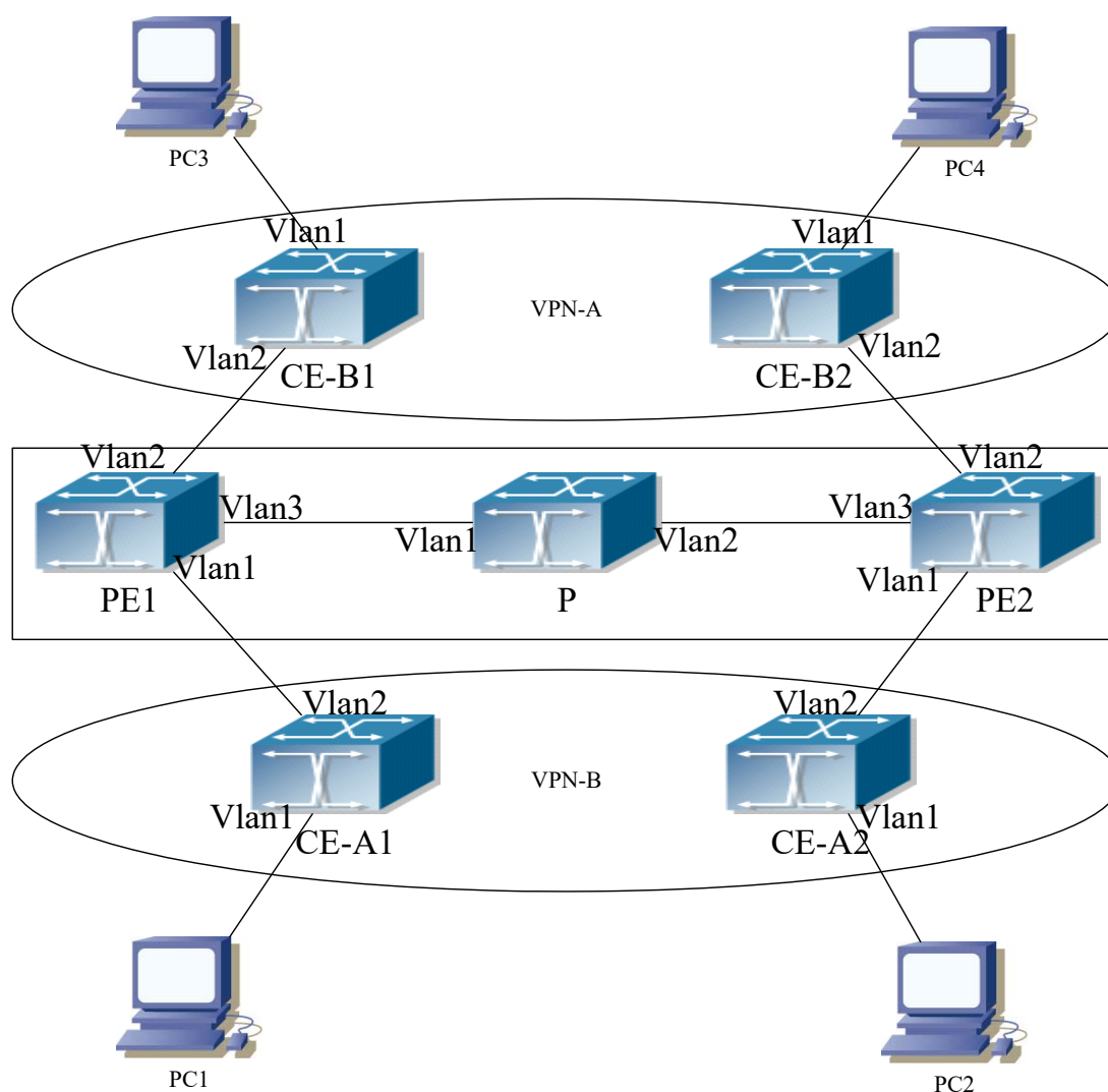
图 5-13 MPLS VPN 典型案例
