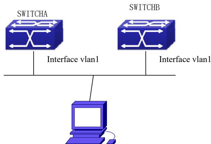
图 8-12 RRP 网络拓扑示意图
