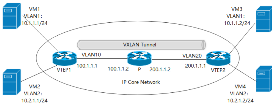
图 12-3 静态 VXLAN 组网
