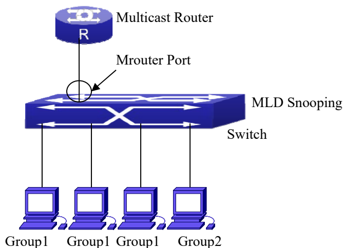
图 13-17 打开交换机 MLD Snooping 功能图
