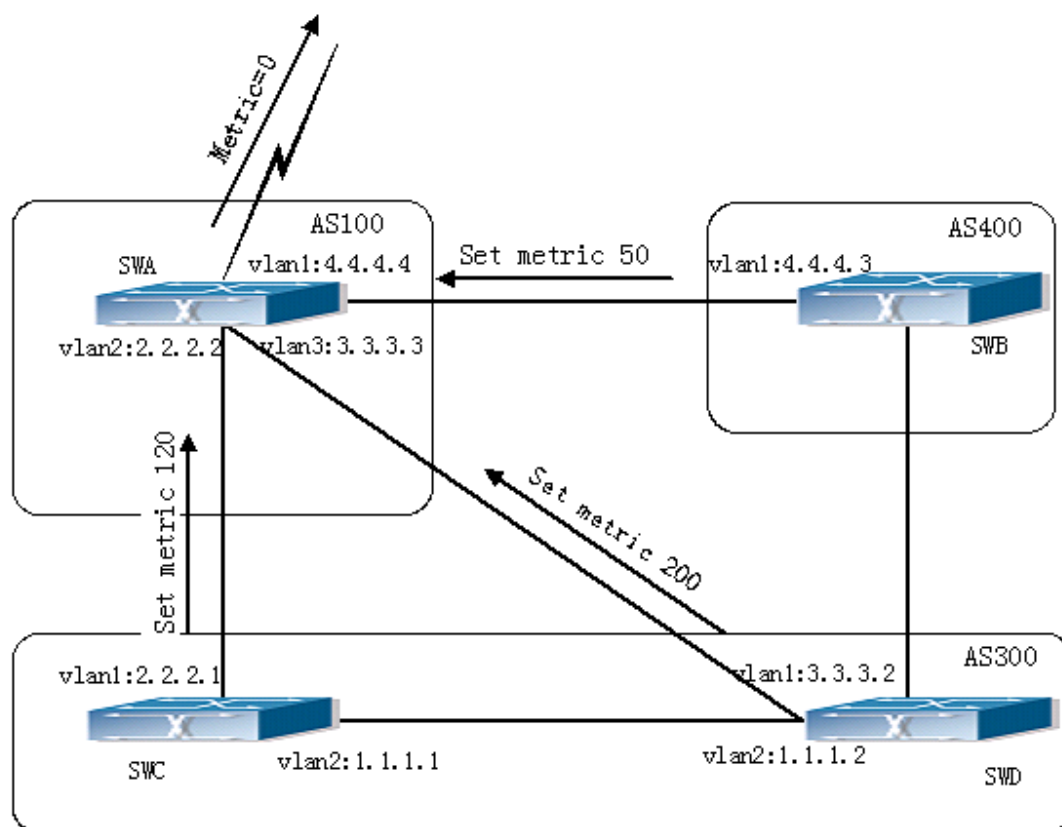
图 5-12 MED 配置拓扑图
