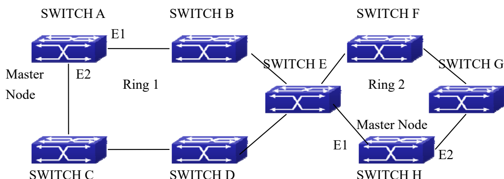
图 8-13 RPP 示意图
