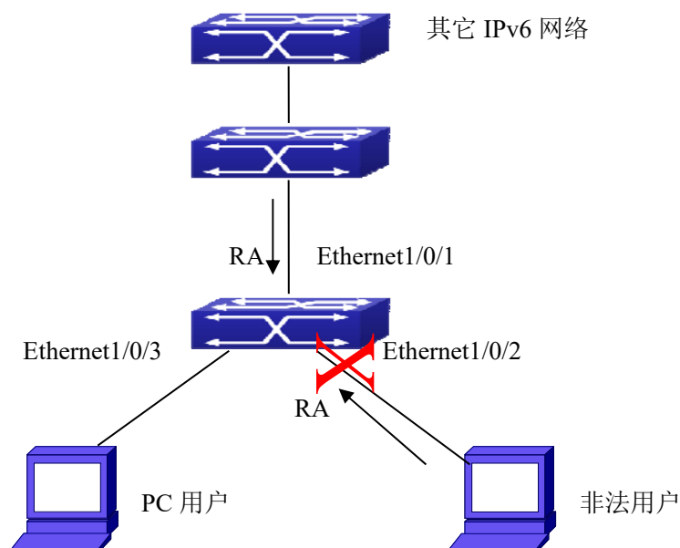
图 13-19 IPv6 安全 RA 案例示意图
