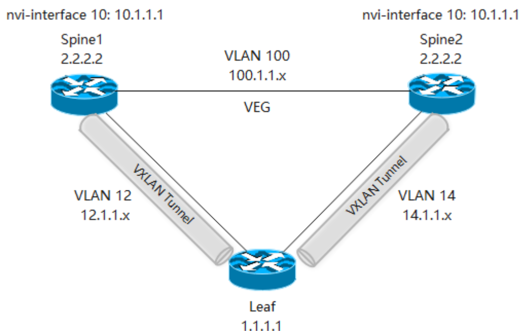
图 13-7 EVPN VXLAN 集中式多活网关
