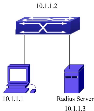
图 7-19 IEEE802.1x 配置举例拓扑图
