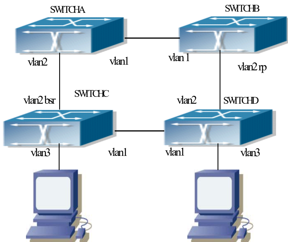
图 6-2 PIM-SM 典型环境
