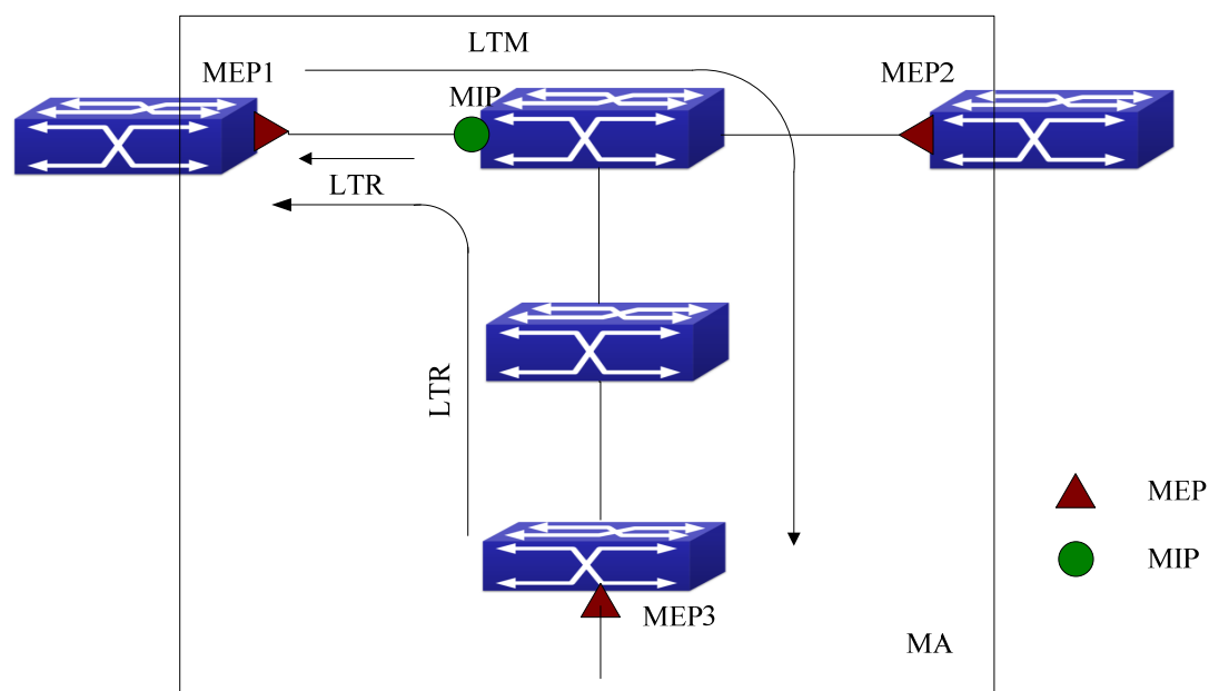
图 3-22 路径发现示意图
