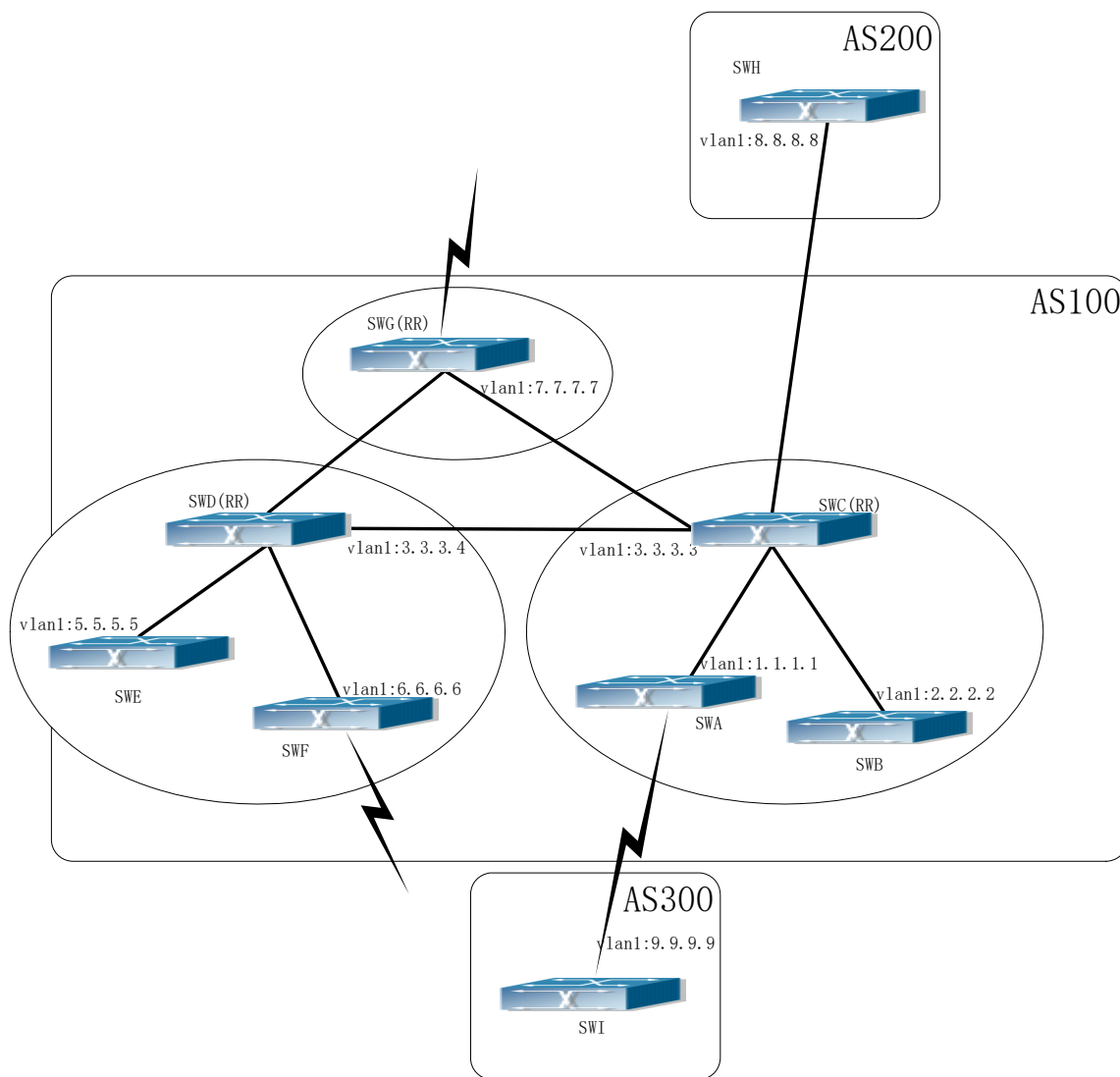
图 5-11 路由反射器拓扑图
