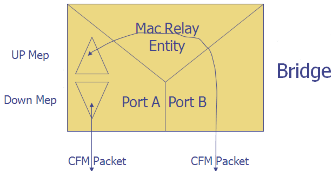
图 3-20 Down MEP 和 Up MEP 区别
