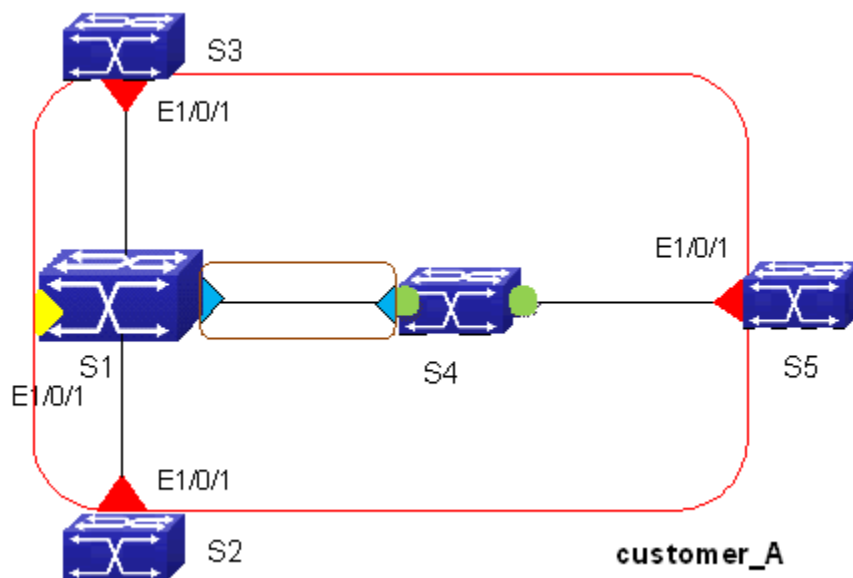
图 3-25 MD, MA, MEP 和 MIP 配置图
