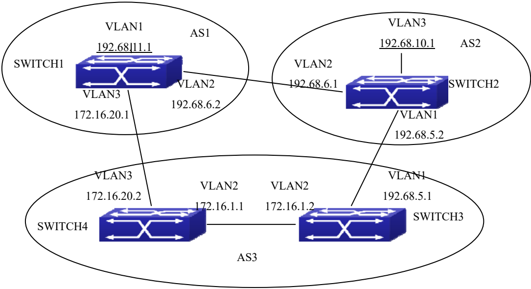
图 5-1 策略路由配置示意图
