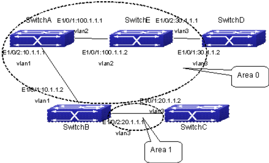
图 5-5 OSPF 自治系统网络拓扑示意图
