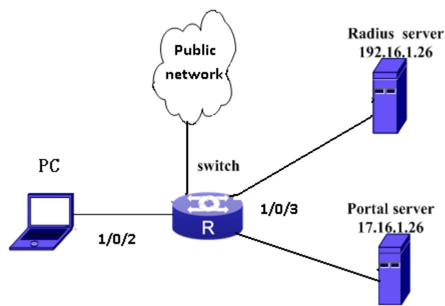
图 7-37 dius server 逃生功能典型案例
