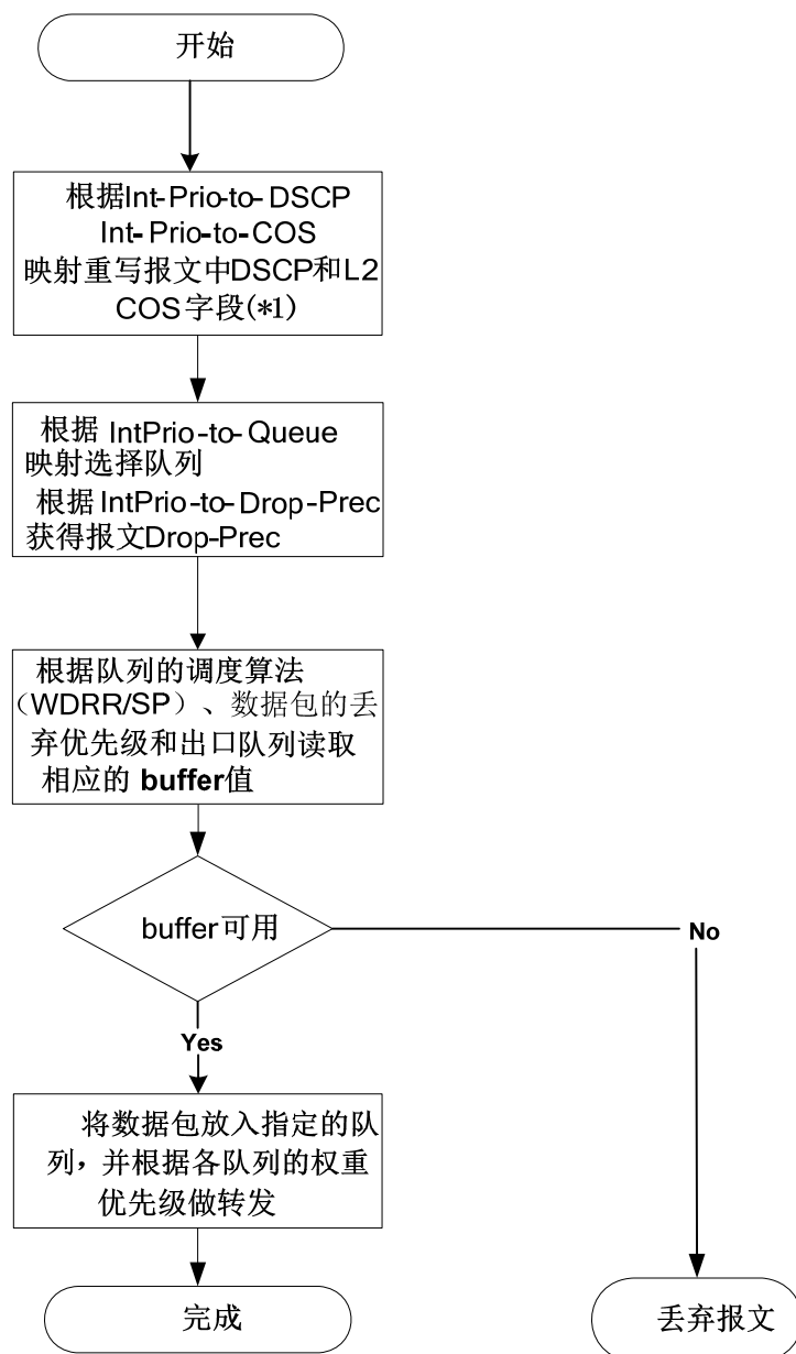
图 7-43 整形和排程流程
