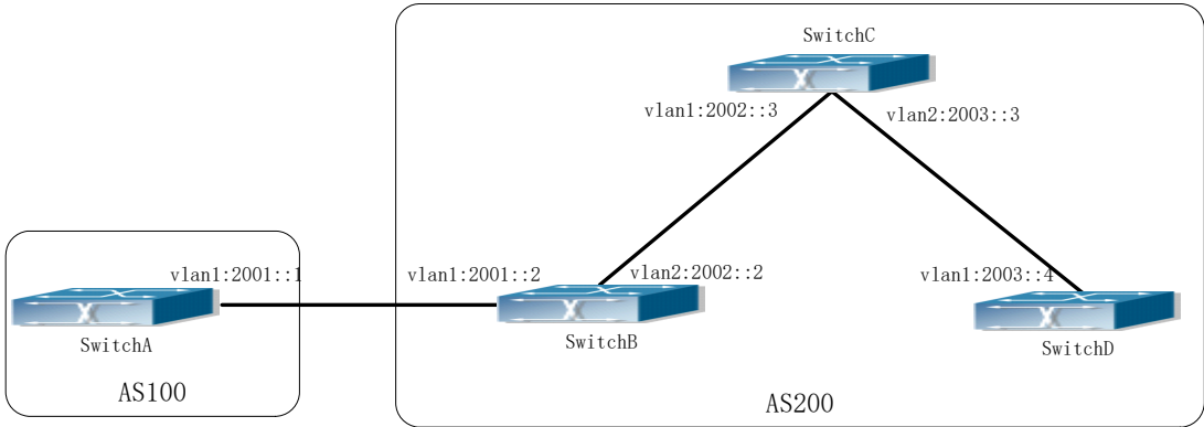
图 13-10 BGP 网络拓扑图
