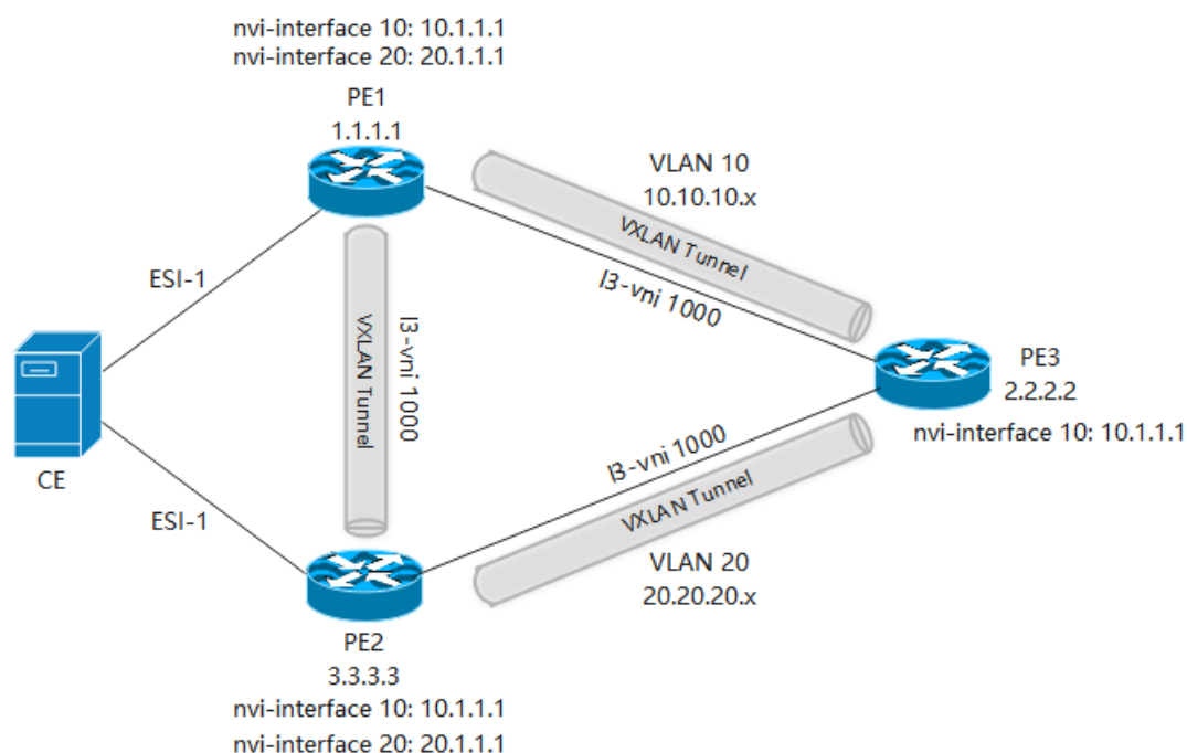
图 13-8 EVPN 双归接入 (VXLAN)
