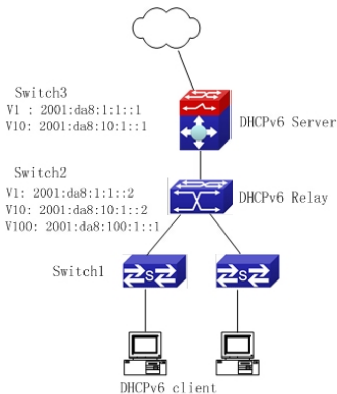
图 13-6 DHCPv6 relay option 示意图
