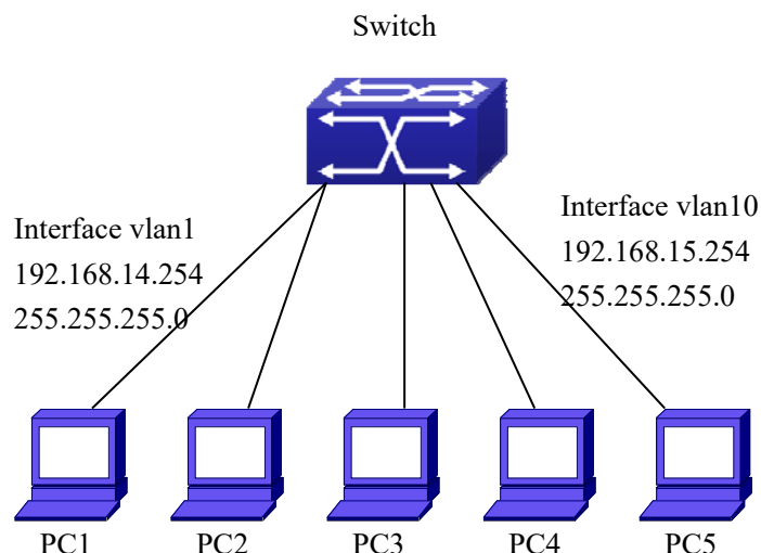
图 4-12 免费 ARP 发送功能配置案例
