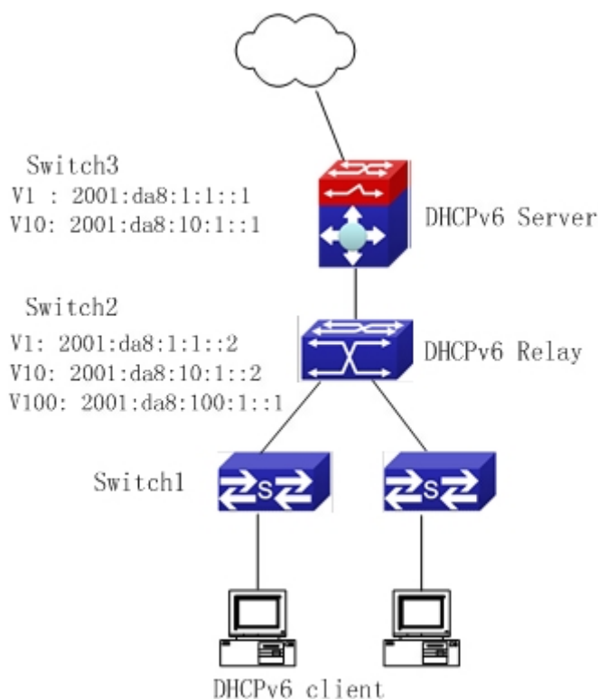
图 13-2 DHCPv6 配置举例示意图 1
