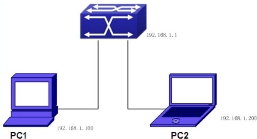
图 4-9 Arp local proxy 功能示意图
