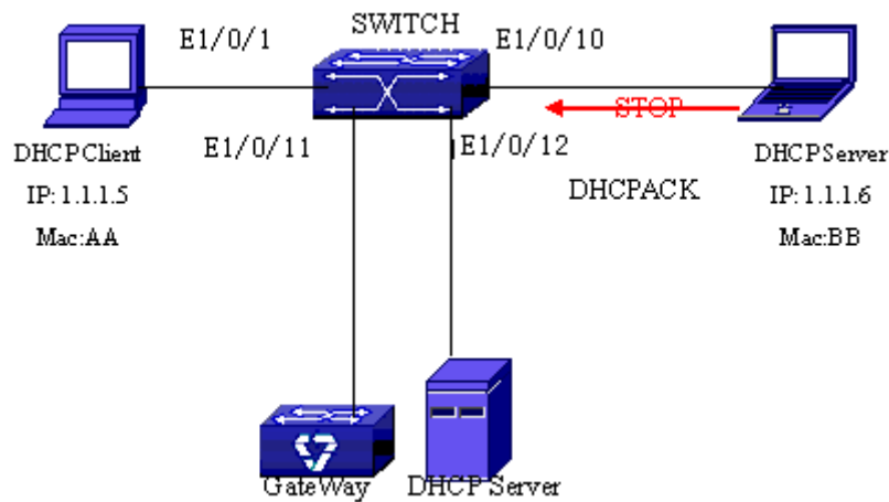
图 4-20 DHCP Snooping 防止非法 dhcp server 示意图
