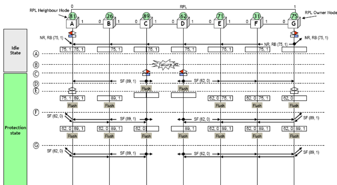
图 8-6 链路故障
