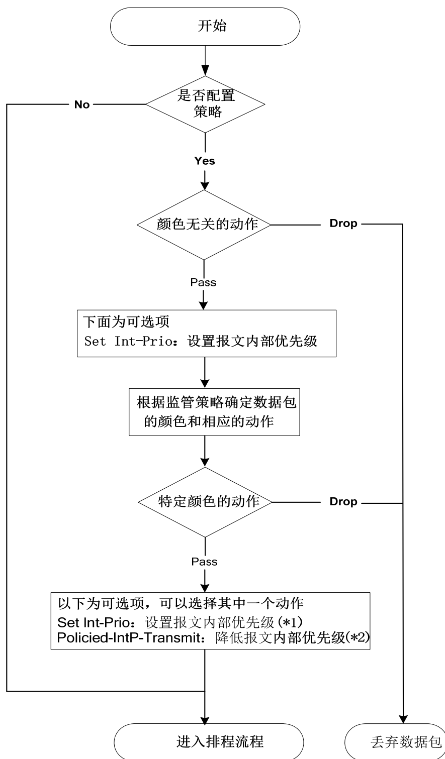
图 7-42 监管和重写流程
