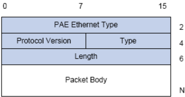
图 7-3 EAPOL 数据包格式
