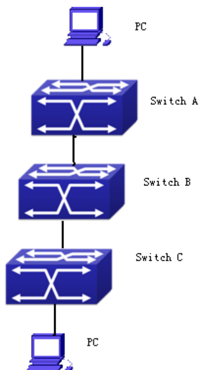
图 3-30 GVRP 典型应用拓扑图
