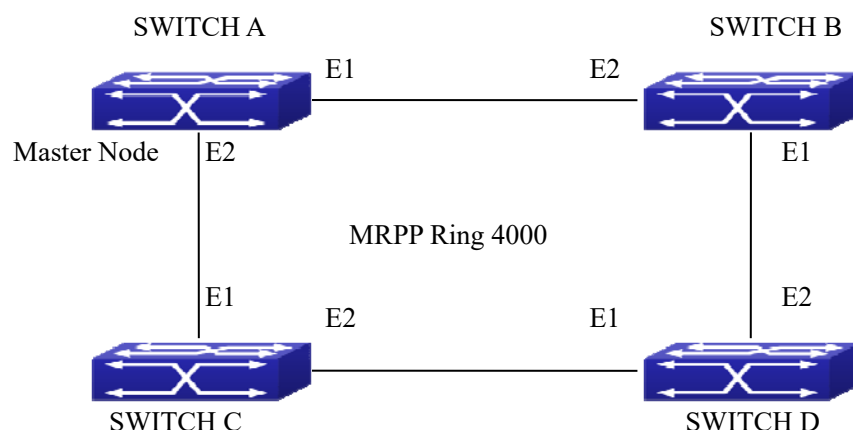
图 8-14 RPP 典型配置案例
