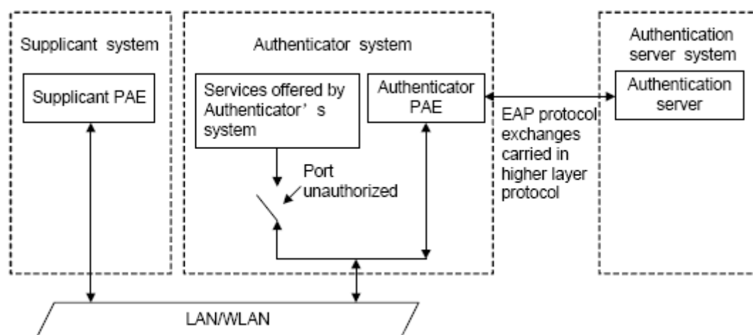
图 7-1 802.1x 认证体系结构
