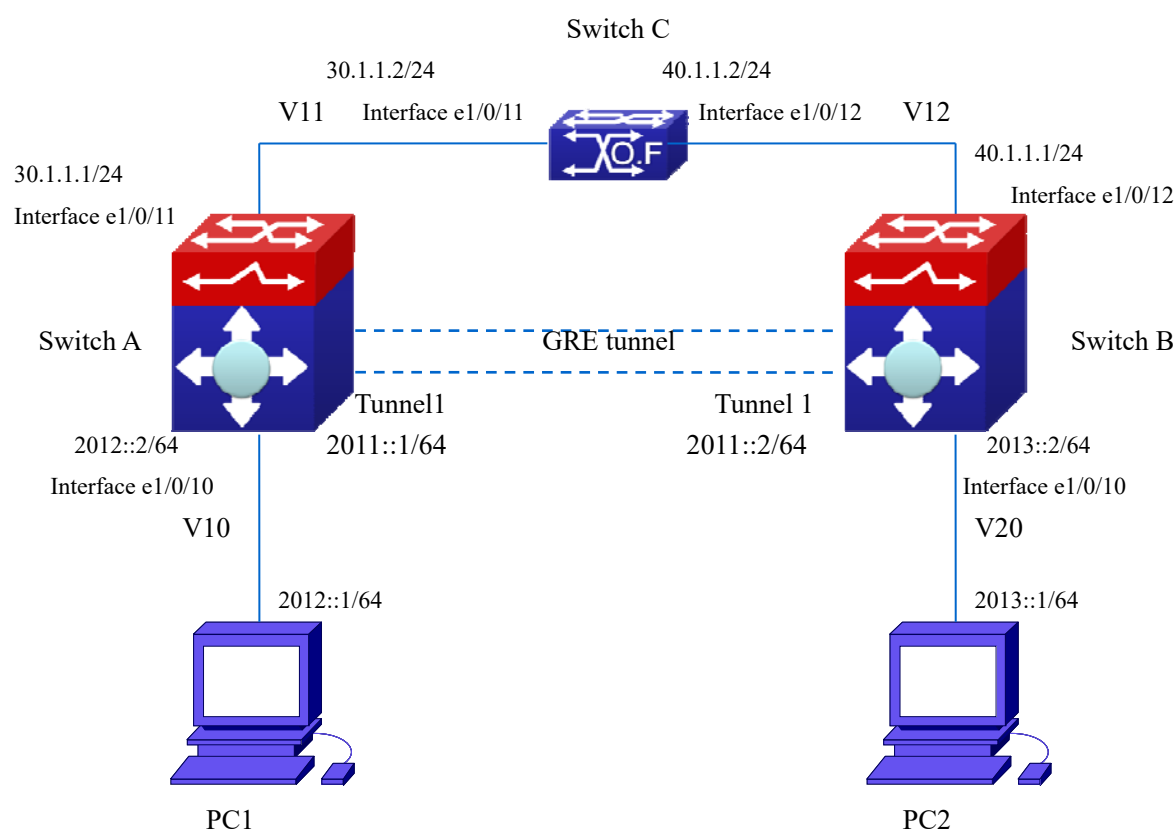
图 5-16 GRE 隧道引用业务环回组典型配置组网图
