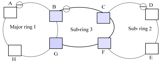
图 8-10 虚通道的交叉环拓扑
