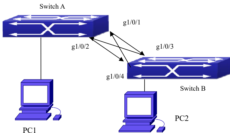
图 3-6 光纤交叉连接
