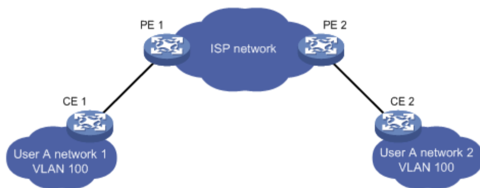
图 3-14 BPDUs Tunnel 应用环境
