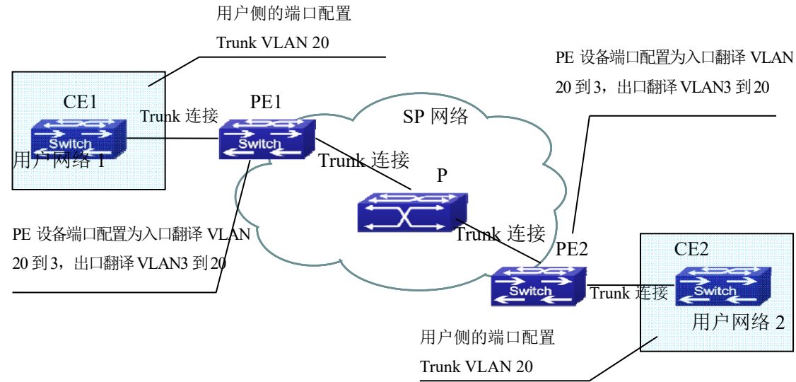
图 3-32 VLAN-translation 典型应用拓扑
