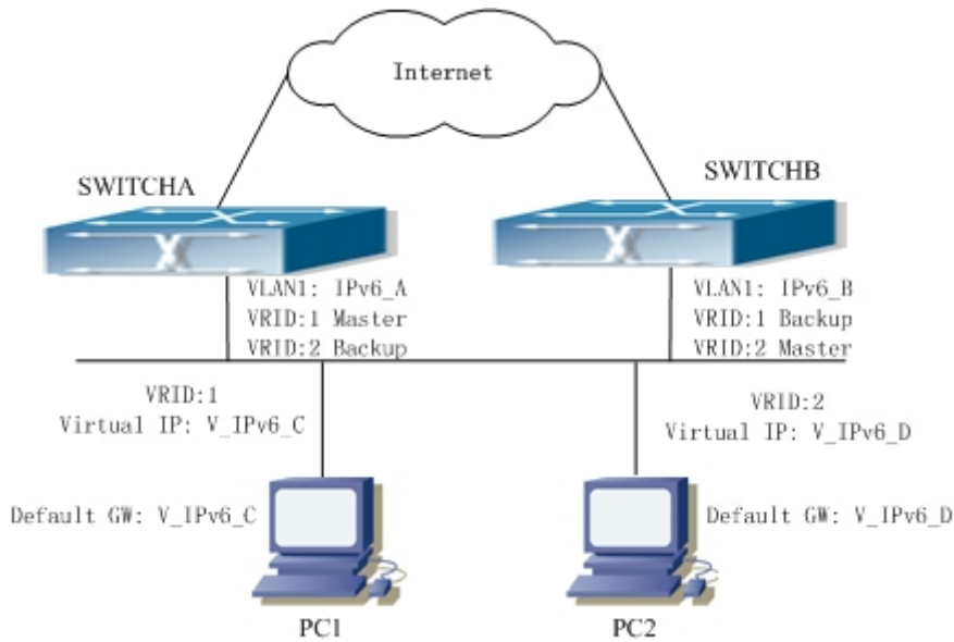
图 13-22 RRPv3 典型网络拓扑
