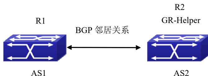
图 5-23 GR 的应用环境
