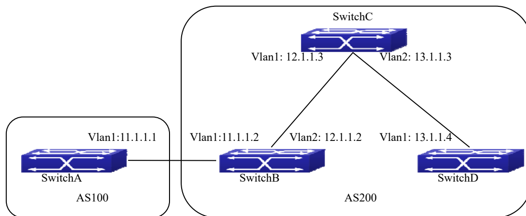
图 5-9 BGP 网络拓扑图
