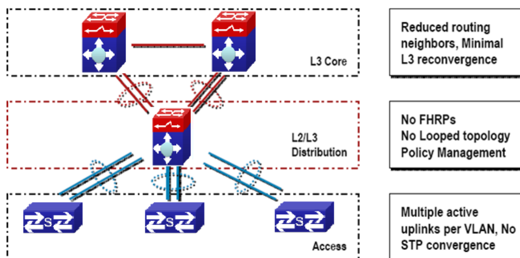
图 11-3 用虚拟化技术的企业网
