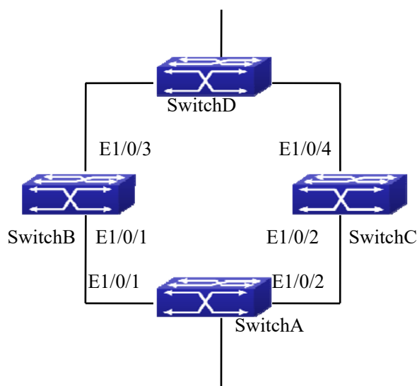
图 8-20 LSM 典型配置案例
