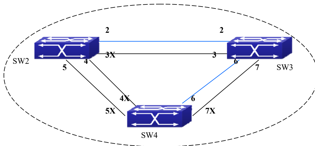
图 8-4 MSTP 变更后 MSTP 域内实例 3 的拓扑
