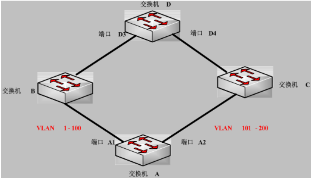
图 8-16 LAN 负载均衡
