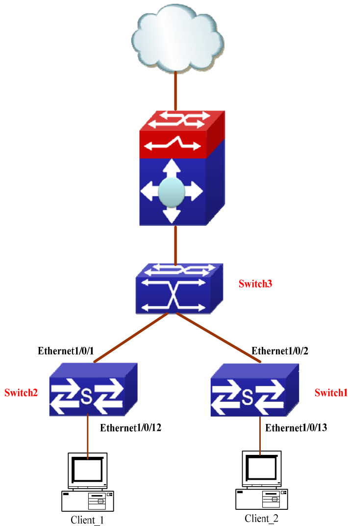
图 13-20 AVI 功能典型的应用网络拓扑环境
