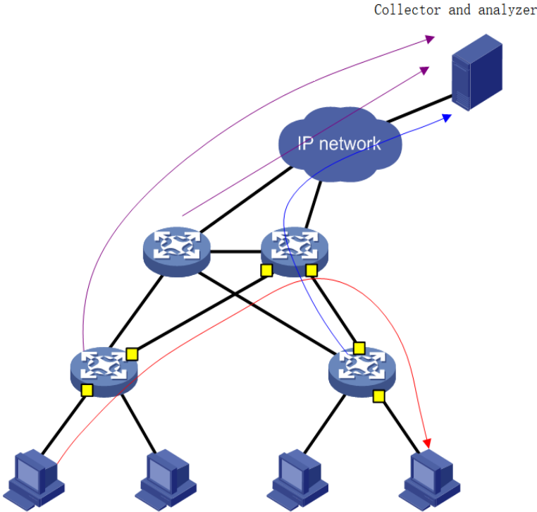
图 13-19 Telemetry 典型网络模型
