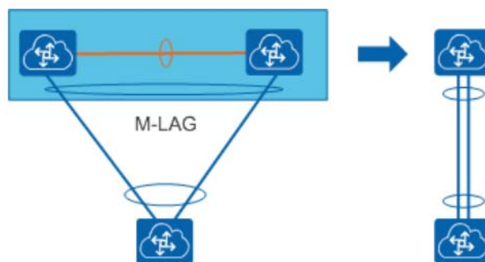
图 13-10 MC-LAG示意图
