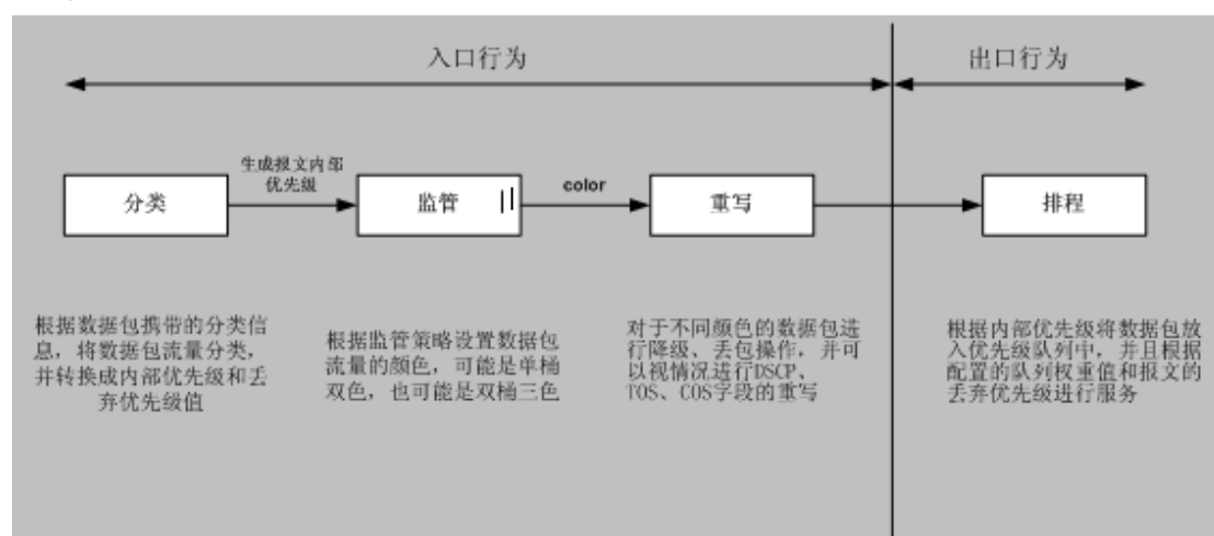
图 7-40 QoS 基本模型
