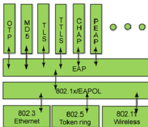
图 7-8 EAP 认证方法协议栈
