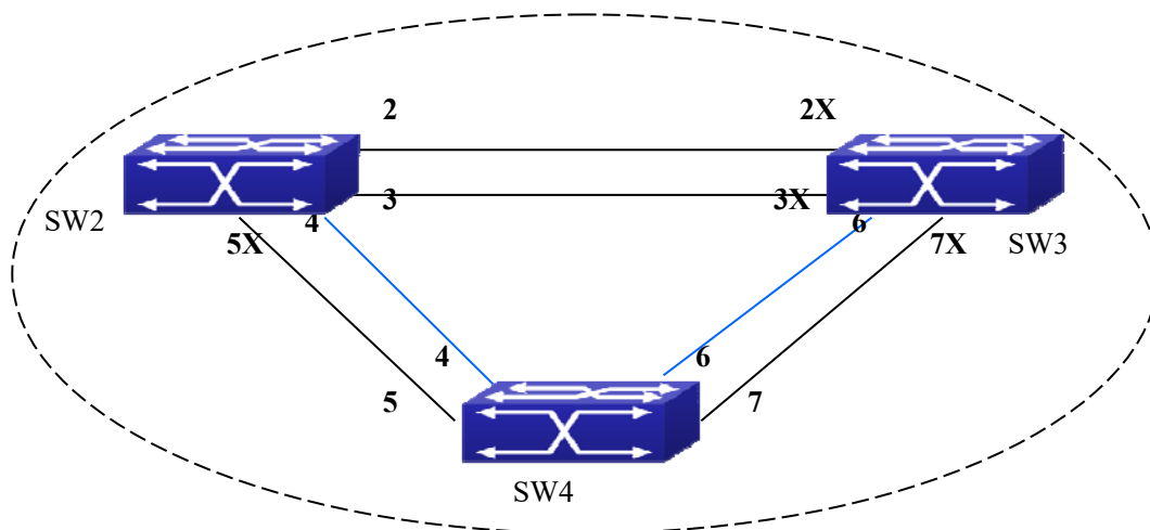
图 8-5 TP 变更后 MSTP 域内实例 4 的拓扑
