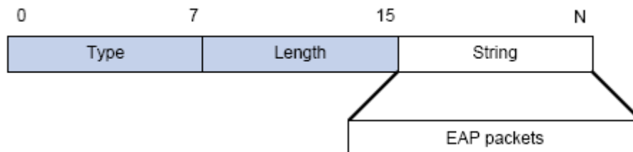
图 7-6 EAP-Message 属性封装
