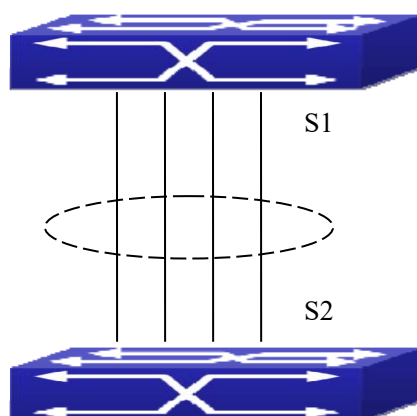
图 3-10 以 LACP 方式配置 Port Channel
