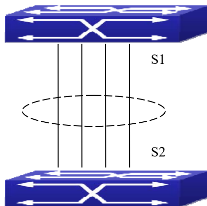
图 3-11 以 ON 方式配置 Port Channel
