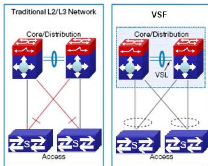
图 11-2 SF 示意图
