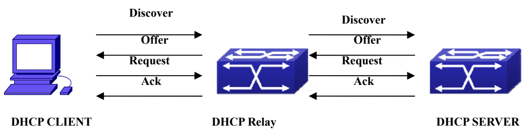
图 4-15 DHCP 中继
