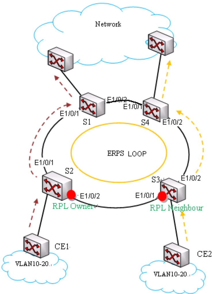
图 8-11 RPS 的配置应用
