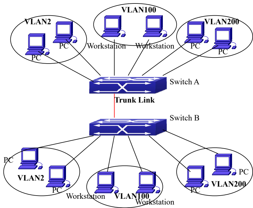
图 3-27 VLAN 典型应用拓扑图
