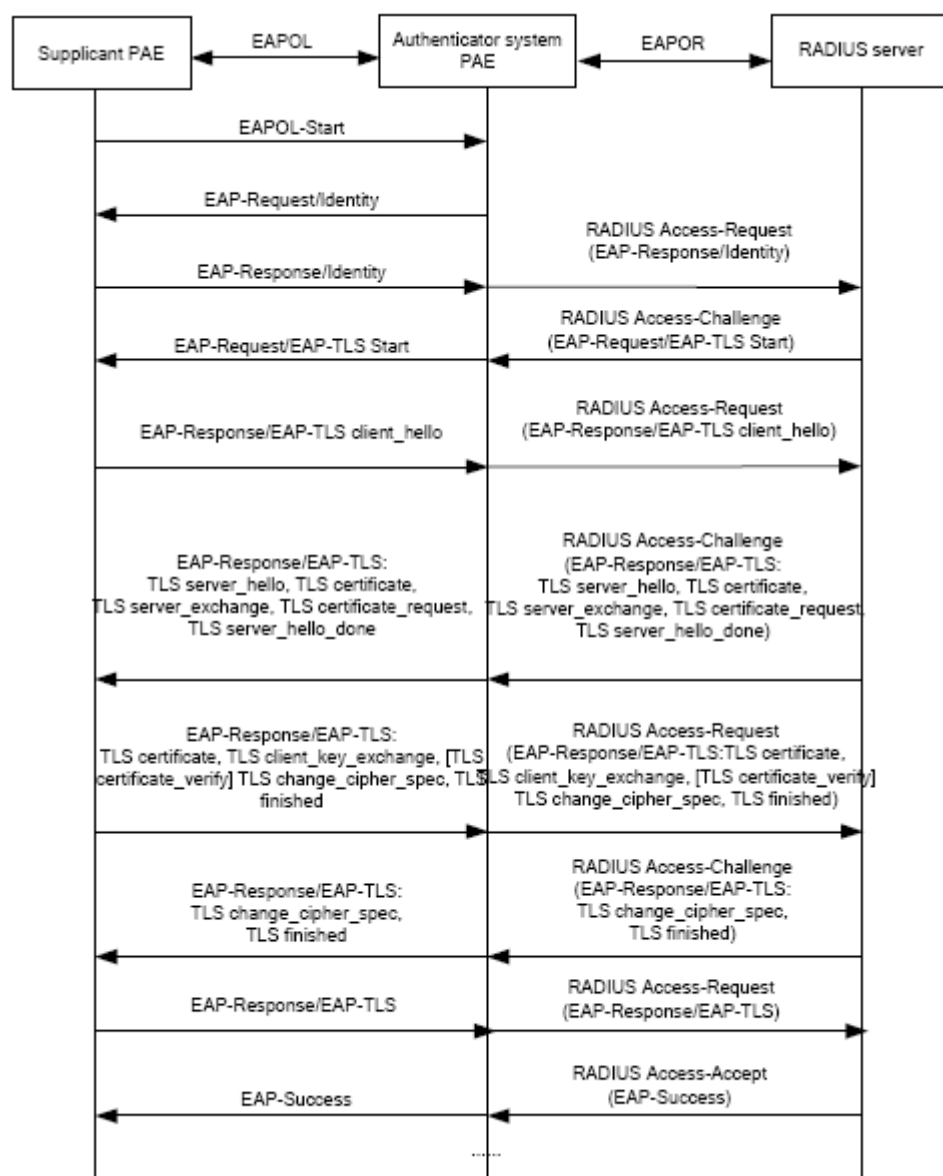
图 7-10 802.1x EAP-TLS 认证流程
