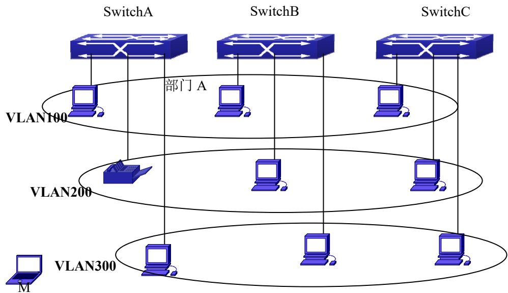
图 3-33 动态 VLAN 典型应用拓扑
