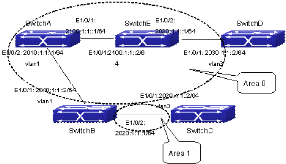
图 13-9 OSPFv3 自治系统网络拓扑示意图
