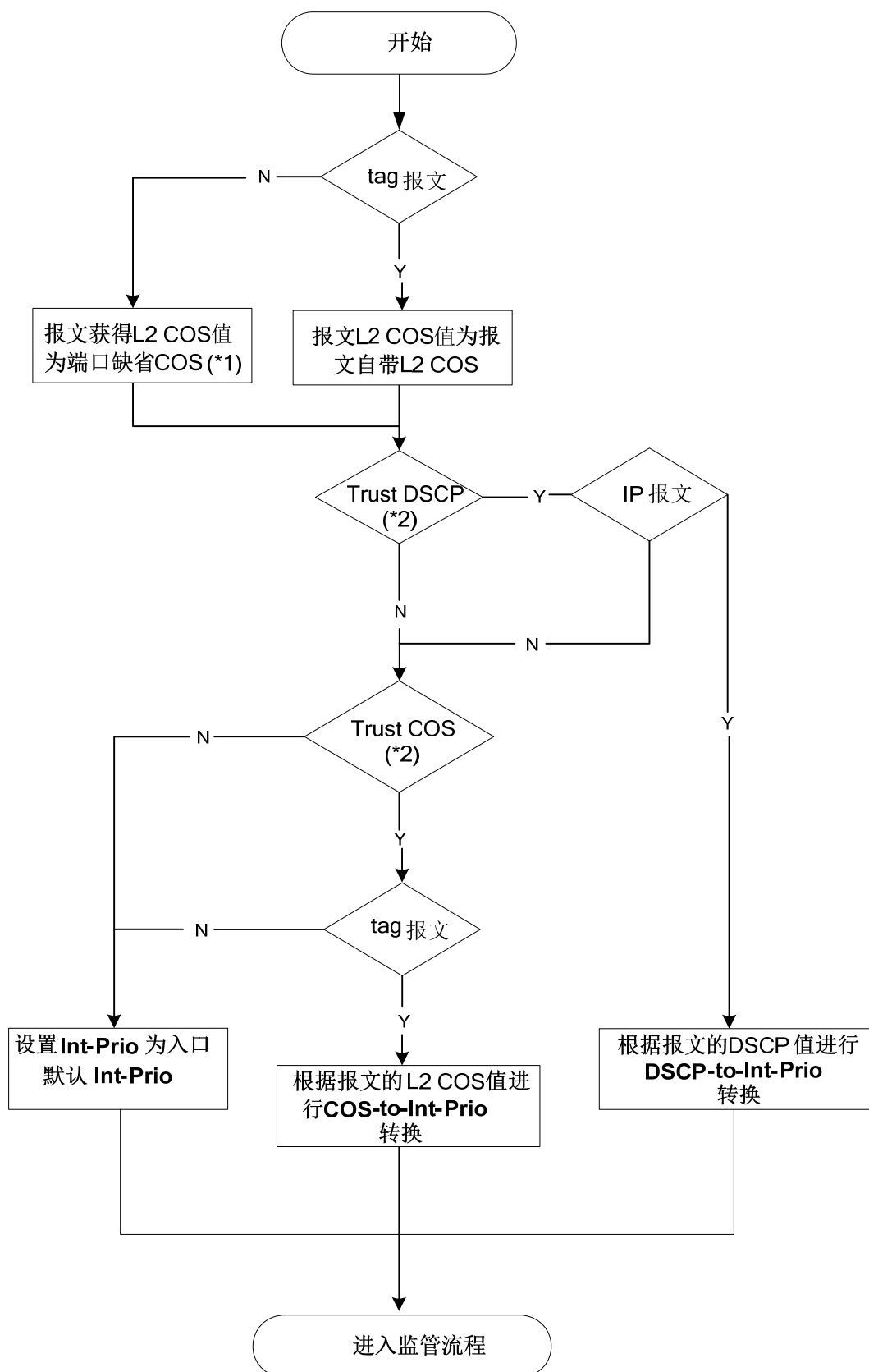
图 7-41 分类流程
