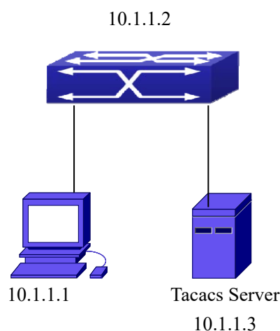
图 7-23 TACACS+配置示意图
