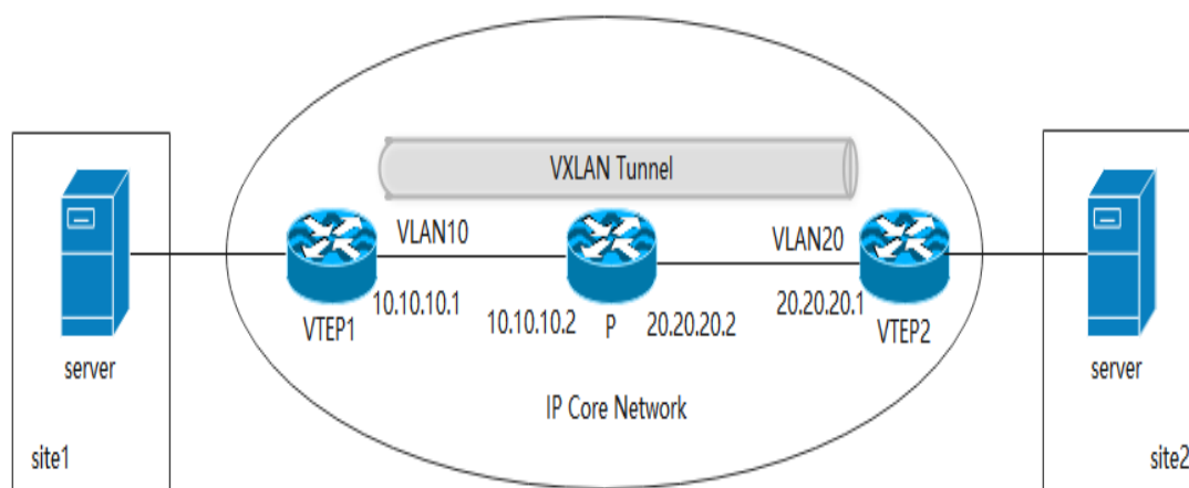
图 13-4 EVPN VXLAN 二层互通组网图
