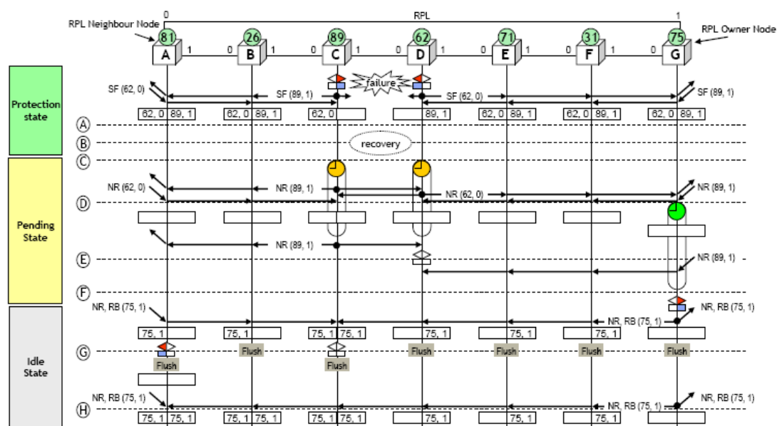
图 8-7 链路可逆倒换方式故障恢复
