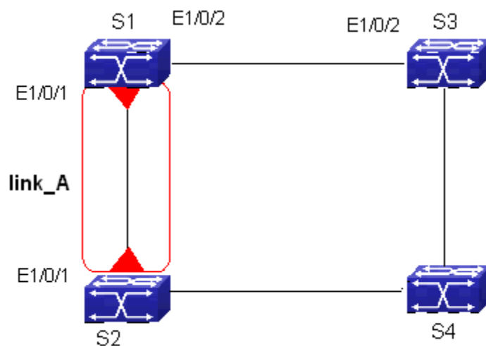
图 3-24 ULPP 联动配置图
