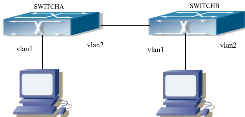
图 13-12 PIM-DM 典型环境
