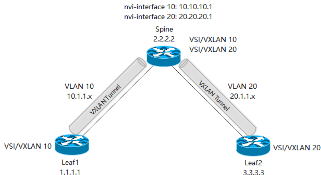
图 13-5 EVPN VXLAN 集中式网关
