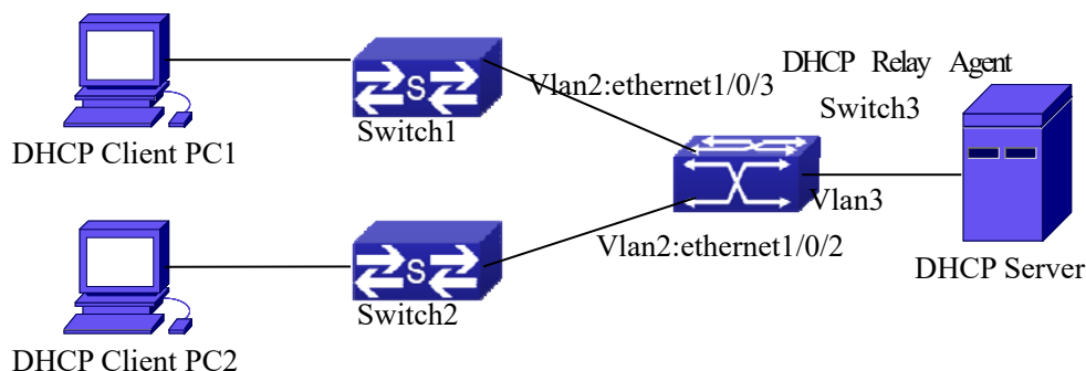
图 4-19 DHCP option 82 典型应用案例
