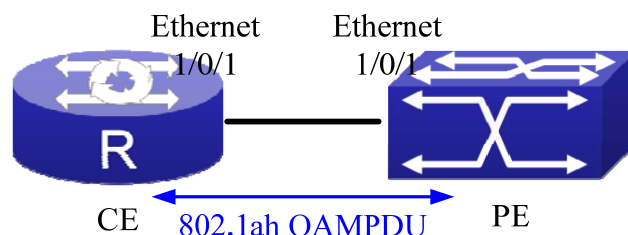
图 3-17 OAM 典型应用拓扑图
