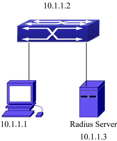
图 7-25 EEE802.1x 配置举例拓扑图
