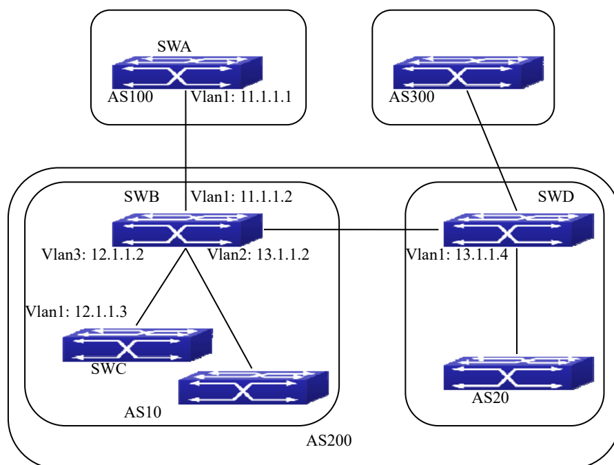
图 5-10 联盟配置拓扑图
