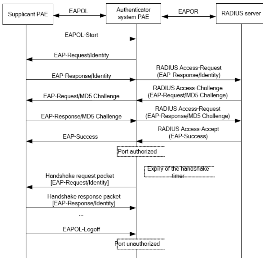
图 7-9 802.1x EAP-MD5 认证流程
