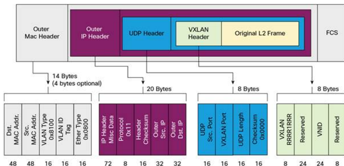
图 12-2 VXLAN 报文封装格式
