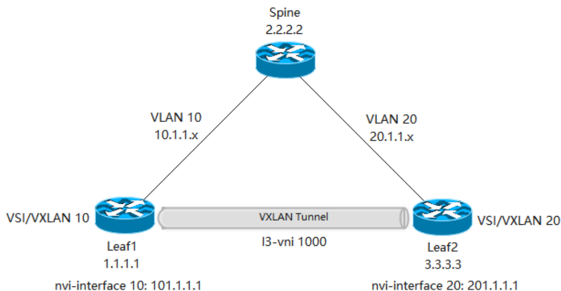
图 13-6 EVPN VXLAN 分布式网关
