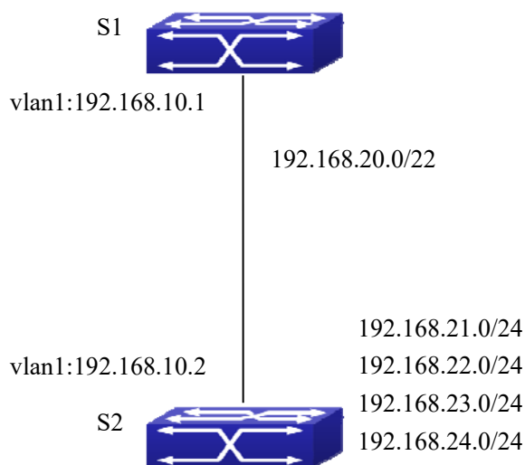
图 5-4 RIP 路由聚合典型应用环境
