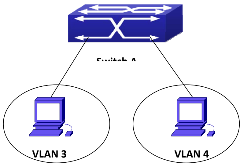
图 3-38 supervlan 典型应用拓扑图
