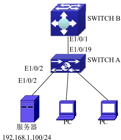
图 4-6 防 ARP 扫描典型配置案例
