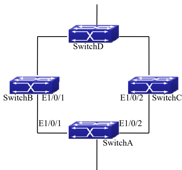
图 8-17 PP 典型配置案例 1
